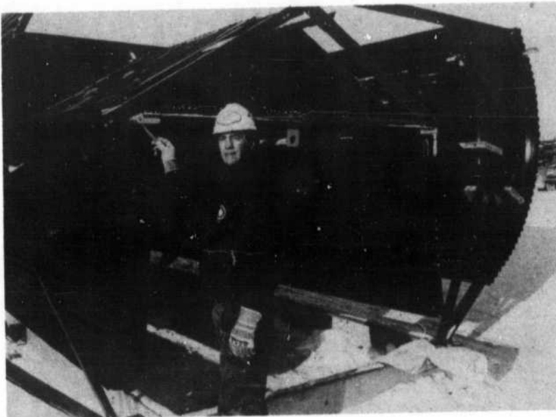
Une fois assemblés au sol par les ferblantiers, ces aérateurs sont hissés au sommet de la bâtisse par une grue de 120 tonnes. M. Yvan Bergeron, délégué de chantier local 116, inspecte une dernière fois le mécanisme de l'aérateur avant sa mise en place. (Photo: Les Communications Gabriel)
