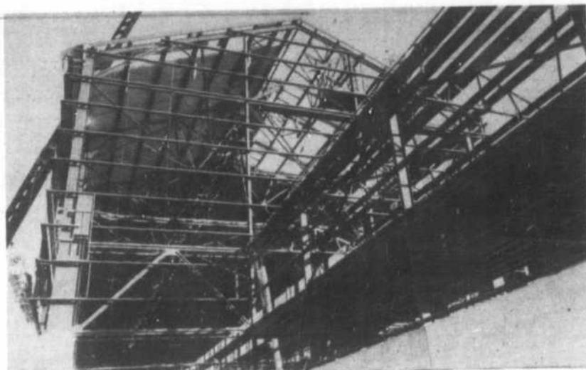
Le travail des ferblantiers consiste à recouvrir les structures d'acier de revêtement d'aluminium. Sur le chantier de la troisième série de cuves d'électrolyse A.B.I., l'installation des aérateurs sur le toit se fait à une hauteur de 65 pieds. (Photo: Les Communications Gabriel).
