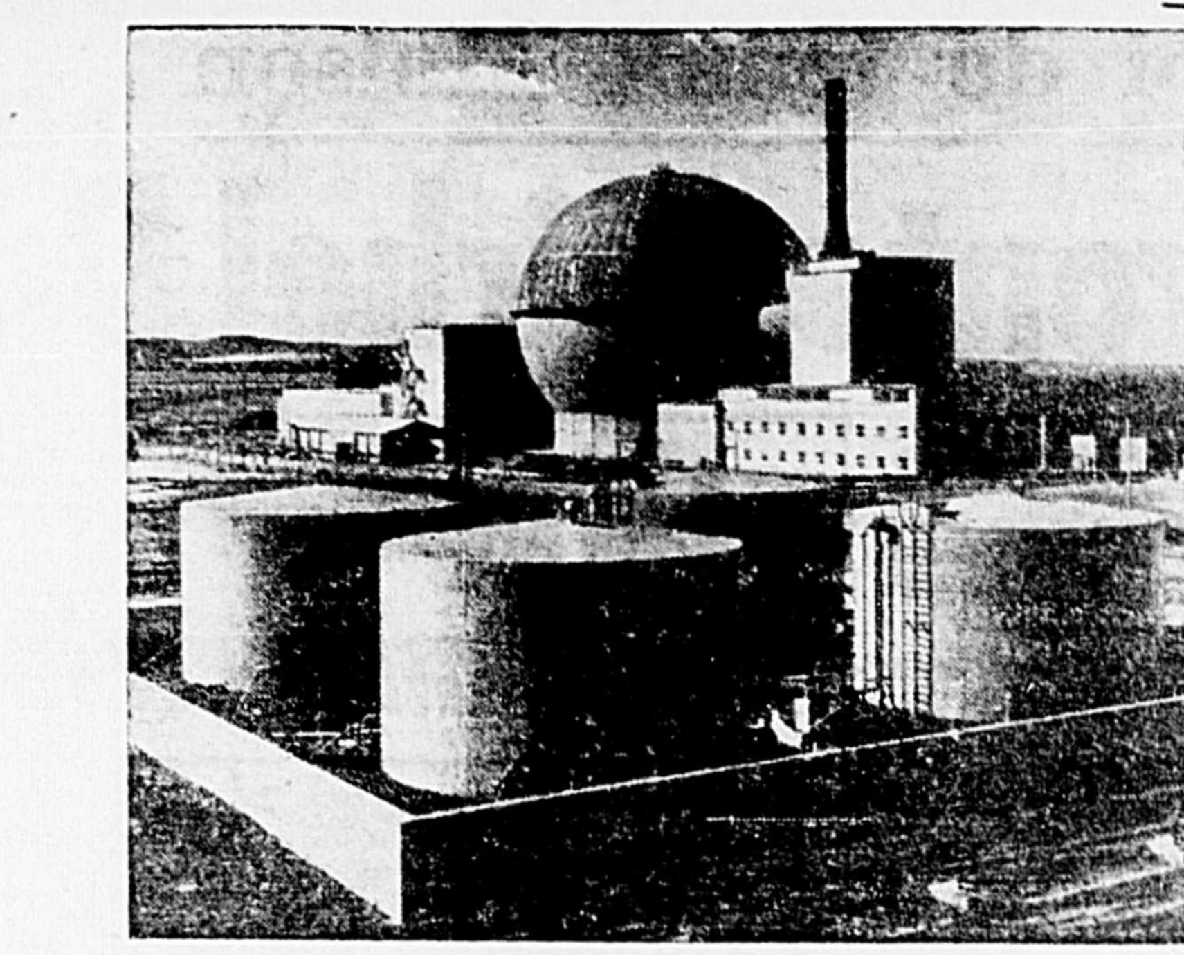
Les autorités de l'Energie Atomique de Grande-Bretagne ont érigé un réacteur-reproducteur à fissilité rapide capable de produire 60 MW de chaleur dans le centre d'un réacteur pas plus grand qu'une boîte. La sphère contenant le réacteur-reproducteur est photographiée ici avec des réservoirs d'huile au premier plan. Le réacteur est une partie d'un établissement de recherches et de développement construit par les autorités de Douvres au nord des Iles Britanniques.
