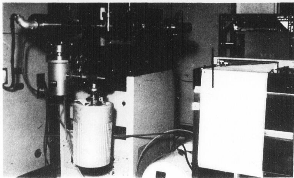
Spectromètre de masse magnétique de haute résolution. Equipé d'un système à ultravide [on y retrouve 10000 milliards de molécules de moins que dans l'atmosphère terrestre] l'appareil a été conçu pour effectuer l'analyse isotopique de différents éléments en faible quantité et fournir ainsi un moyen de déterminer l'origine de certains constituants alimentaires. Cet appareil découlant de la haute technologie est une réalisation québécoise.
