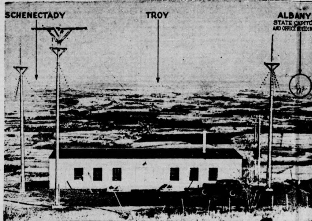
Ce poste de télévision, en construction sur les monts Helderberg, à 12 milles de Schenectady, (N.-Y.) sera le plus puissant des États-Unis avec une force de 10 kilowatts.
