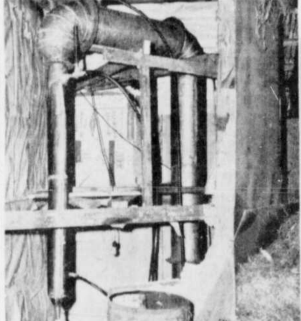
LA COLONNE — C'est goutte à goutte, que l'alcool frelaté s'achemine, de la bouilloire, au réservoir, en passant par la colonne. Cette photo nous montre cette dernière, du moins sa partie qui était au deuxième étage de la grange, parmi le foin et la paille.
