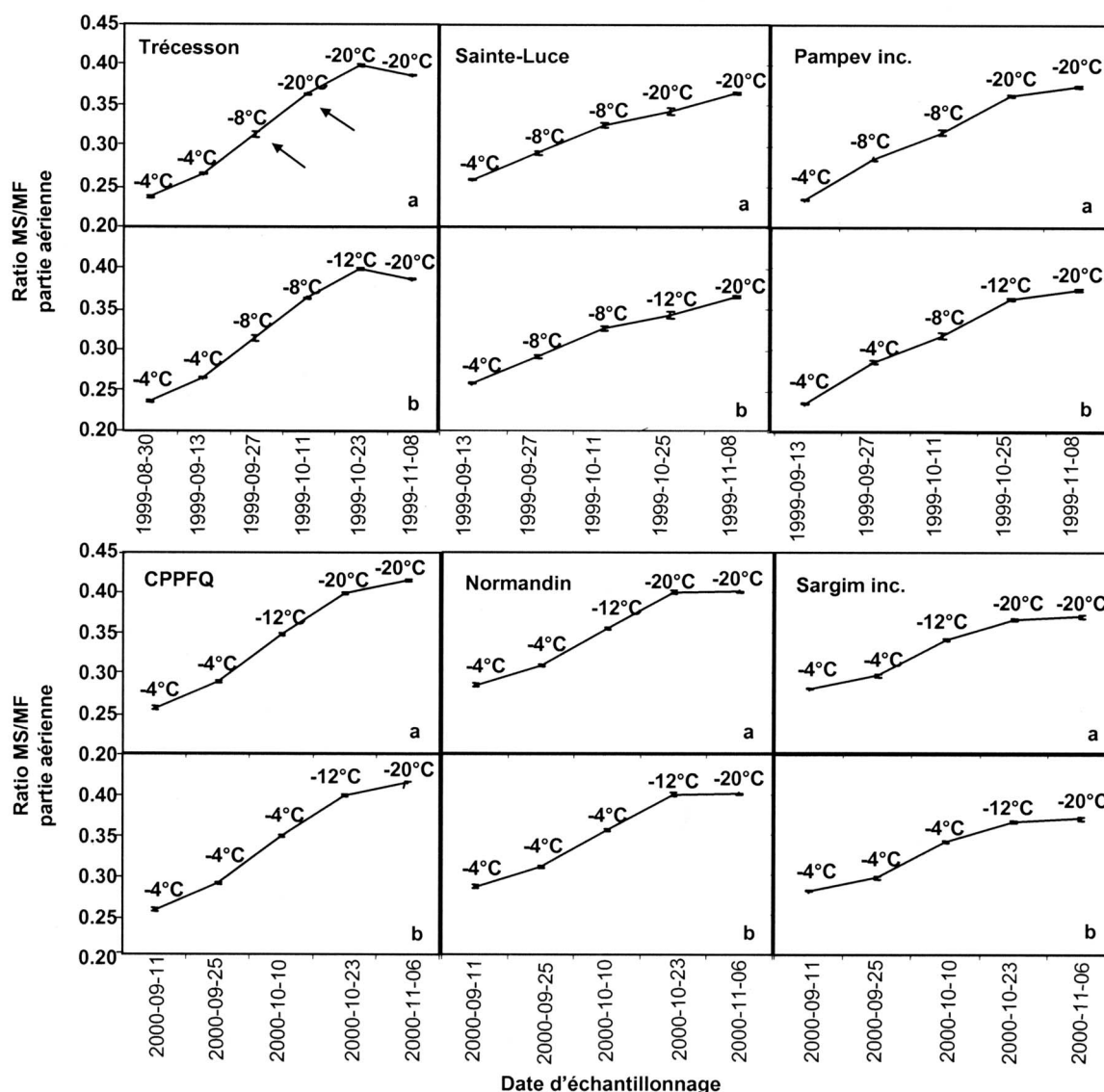
Figure 13. Évolution des seuils de tolérance au gel, dans chacune des six pépinières, spécifiques : a) aux parties aérienne et b) aux racines des plants d'épinette blanche (1+0). Les flèches indiquent que des taux d'acquisition quotidiens de tolérance au gel des plants peuvent être déduits des pentes ( 0^{\circ}\text{C}/\text{jour} ) propres aux seuils de tolérance, calculés entre deux dates consécutives d'échantillonnage.
