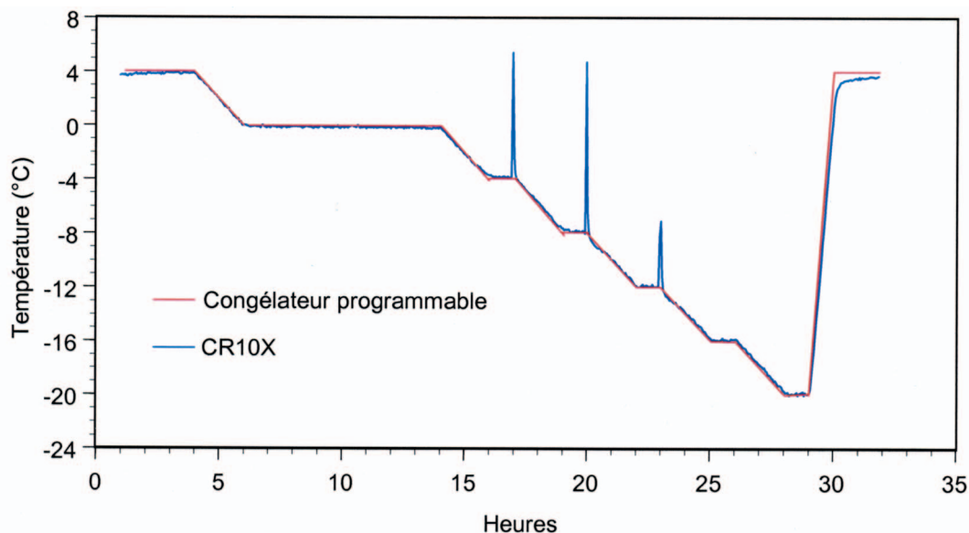
Figure 3. Exemple d'un cycle de congélation illustrant les températures à atteindre (trait en rouge), ainsi que le maintien constant de chaque température-cible sous forme d'un « palier », durant une heure. Pour confirmer l'atteinte des températures simulant les gels artificiels, un suivi continu de l'évolution de la température, à intervalle de trois minutes, a été effectué à l'aide d'un système d'enregistrement programmable (CR10X) muni de deux sondes de température (trait en bleu). Les pics indiquent l'ouverture de la porte du congélateur et coïncident avec la sortie des plants une fois que ceux-ci ont subi les différents gels artificiels ciblés ( T_1 = -4 °C, T_2 = -8 °C, T_3 = -12 °C et T_4 = -20 °C).
