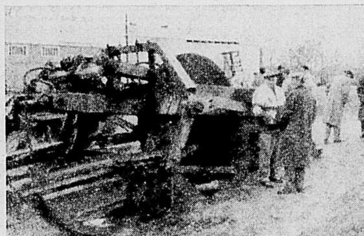
Cette photo illustre bien la grosseur et la puissance des charrues utilisées par le ministère de la Colonisation pour le défrichement de nouvelles terres de l'Abitibi. Ce sont les plus grosses du genre au monde!
