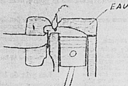
CHEMISE D'EAU AUTOUR DU PISTON
