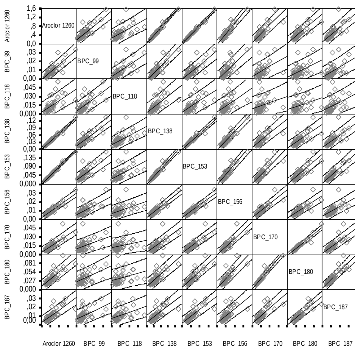
Figure 5.19. Matrice de corrélation entre l'Aroclor 1260 et huit congénères spécifiques de BPC dosés dans les lipides plasmatiques ( \mu\text{g/g} de lipides; intervalles de confiance à 95 % pour les données individuelles). Les coefficients de corrélation de Spearman sont donnés au tableau 5.30.
