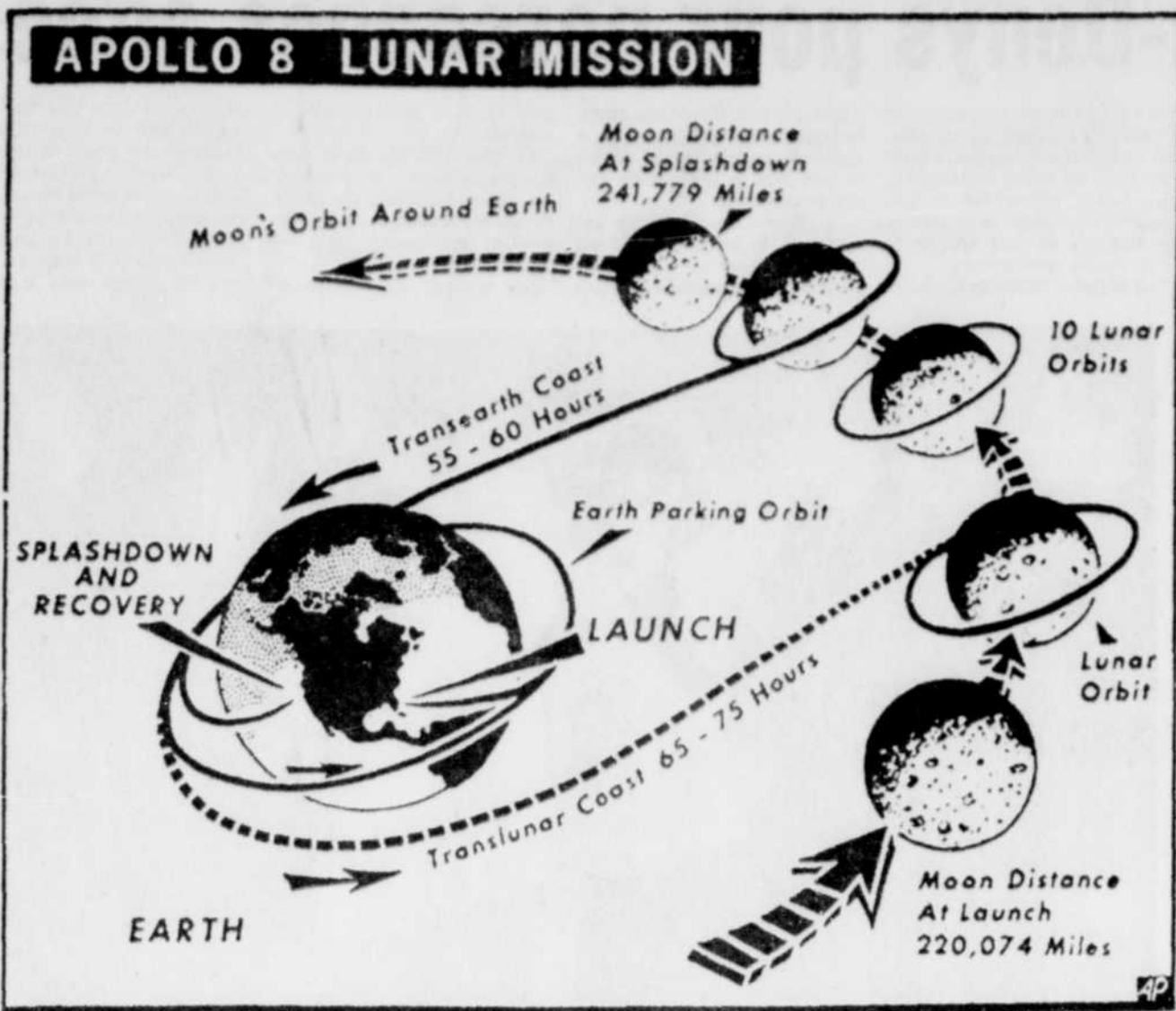
C'EST APPROXIMATIVEMENT LA ROUTE DU vaisseau spatial Apollo 8 de la terre à la lune et de la lune à la terre. Les astronautes du véhicule feront dix tours autour de l'astre qui éclaire les nuits terriennes, avant de revenir vers la terre. Le plus long voyage jamais entrepris par l'homme.
