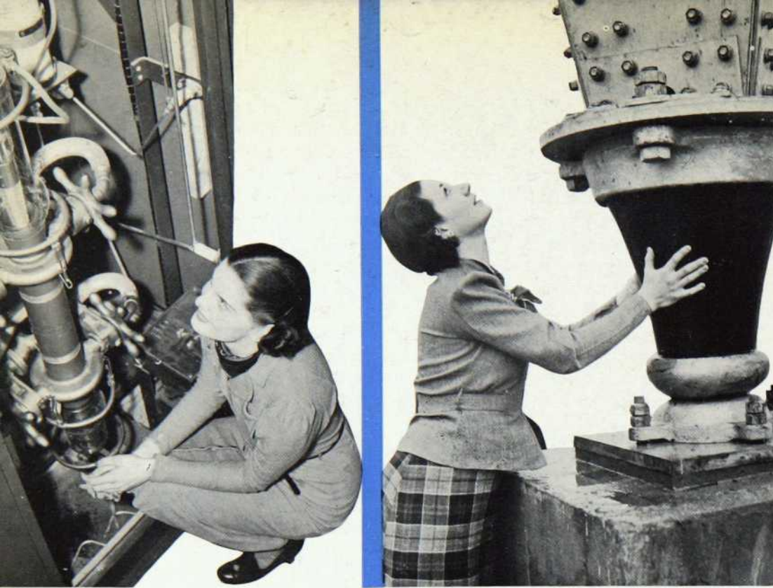
1. A gauche: Une des deux lampes amplificatrices de 100 kilowatts, type 298-A.
