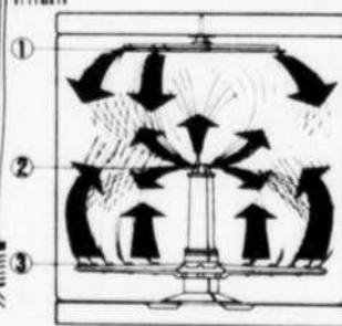
Action de lavage hydrodynamique à 3 niveaux
