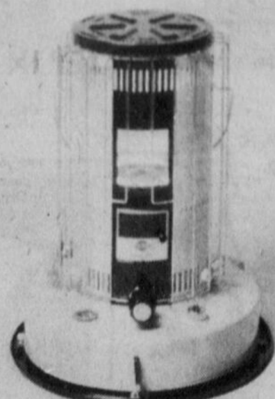
Omni 105: Rendement de 19,500 BTU à l'heure. Idéal pour les pièces et bâtiments de plus grandes dimensions: sous-sols humides, garages, pièces adjucentes, entrepôts, fermes, chantiers de construction. Peut fonctionner pendant 18 heures avec 7.5 litres (1.66 gal.) de kérosène. Hauteur: 559 mm; base de 474 mm. Poids: 12.0 kg.
