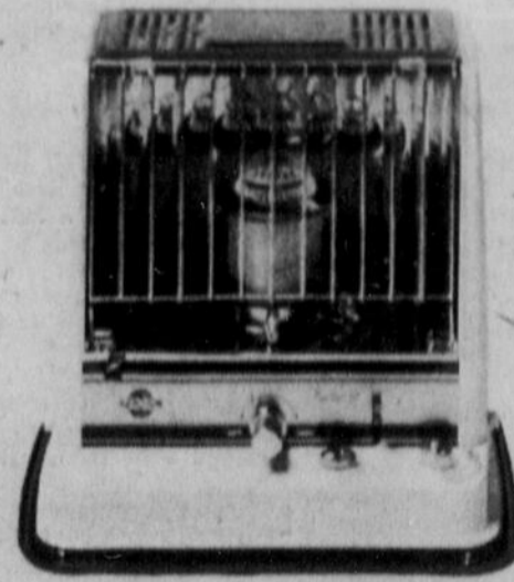
Radiant 10: Rendement de 9,600 BTU à l'heure. Le modèle radiant au kérosène le plus populaire en Amérique. De conception moderne, il s'adapte à tout genre de décor. Peut fonctionner de 27 à 37 heures avec 7.3 litres (1.60 gal.) de kérosène. Hauteur: 485 mm; largeur: 532 mm; profondeur: 387 mm. Poids: 11.2 kg.
