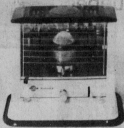
Radiant 8: Rendement de 8,200 BTU à l'heure. Le plus compact et le plus économique de tous les modèles radiants Kero-Sun. Idéal pour chauffer les espaces réduits. Peut fonctionner de 28 à 39 heures avec 5.4 litres (1.42 gal.) de kérosène. Hauteur: 437 mm; largeur: 528 mm; profondeur: 342 mm. Poids: 9.6 kg.
