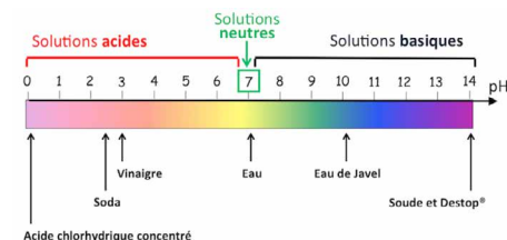
Figure 2 Représentation et exemples de l'échelle du pH. Source : Colas ANSELME, Une pincée d'atomes, [Internet] [Consultée le 13 avril 2022] Disponible à : https://une-pinee-d-atomes.pagesperso-orange.fr/cours-ph/co/l_Acide_basique_ou_neutre.html
