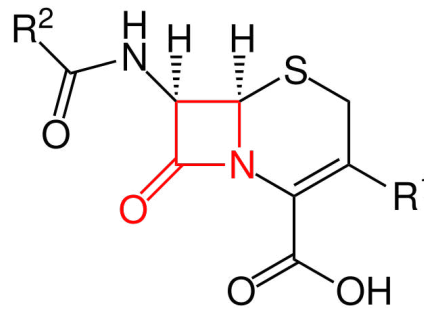
Figure 1 Structure générale d'une céphalosporine. Le cycle \beta -lactame est tracé en rouge, et les éléments R1 et R2 représentent des groupes d'atomes qui varient d'une céphalosporine à l'autre. Source : Jü. Wikimedia commons [Internet]. 2017 [cité 6 avril 2022]. Disponible sur : https://commons.wikimedia.org/wiki/File:Cephalosporines_General_Formula_V1.svg?uselang=fr
