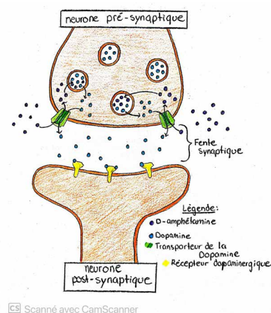
Figure 2 Mécanisme D-amphétamine avec dopamine. Source : Gabriella Marco St-Pierre, dessin, 2022, Vaudreuil.
