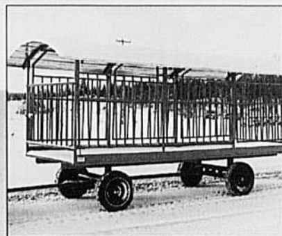
MANGEOIRE POUR INSTALLER SUR WAGON POUVANT PRENDRE 3 BALLES DE 6 x 6 ou 4 BALLES DE 4 PIEDS
