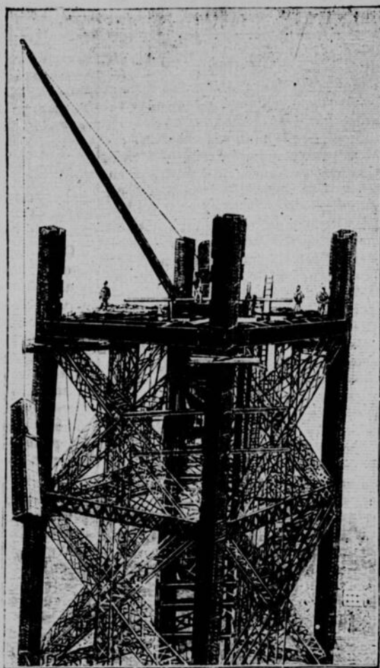
Fig. 2.--Pardessus le deuxième étage. Vue du sommet d'un des piliers sur le point de rejoindre les autres
