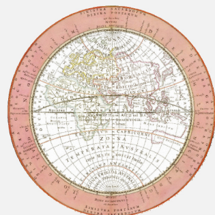
Cellarius, Celestial Atlas Hemisphaerium Orbis Antiqui Cumzonis Circulis et Situ Populorum Diverso
