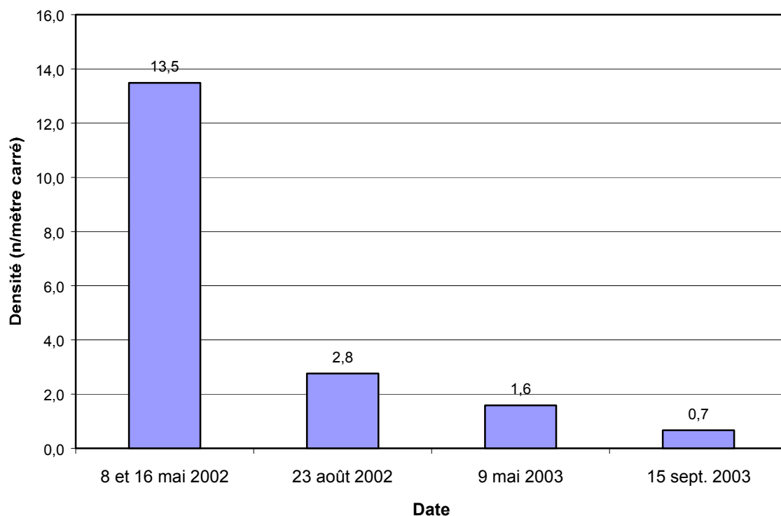
Figure 16.Évolution de la densité de noix viables sur le lit de la rivière du Sud au cours des saisons de récolte 2002 et 2003.
