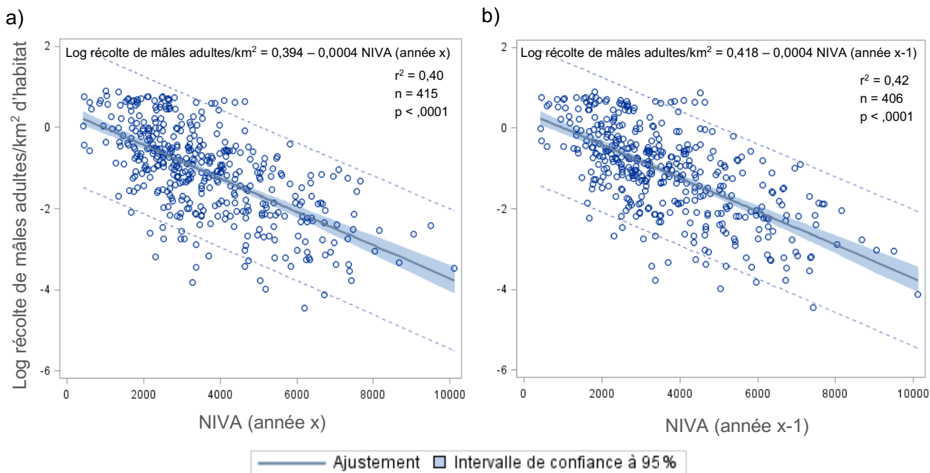
Figure 8. Relation entre la récolte de mâles adultes par kilomètre carré d'habitat dans les différentes zones de chasse (transformée en logarithme) et la rigueur de l'hiver (indice NIVA) évaluée la même année (a) ou l'année précédente (b).
