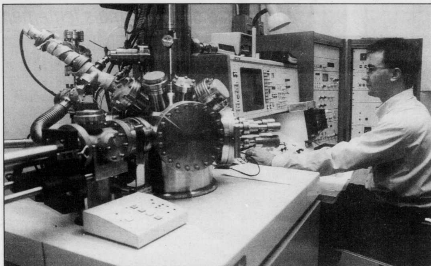
Luc Bélanger se sert d'un microscope Auger, qui peut grossir jusqu'à 300 000 fois, pour analyser des échantillons de métaux placés dans une chambre sous vide. Cet appareil vaut la bagatelle d'un million de dollars.
