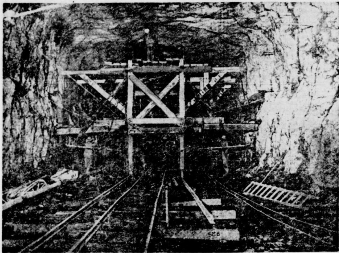
Cette photo nous donne une idée de l'entreprise gigantesque qu'a représentée le percement du tunnel sous le mont Royal, par les chemins de fer nationaux. Ce passage a été foré en deux tronçons par autant d'équipes qui se sont attaquées à la montagne, chacune de son côté.
