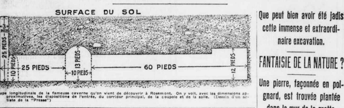
Coupe longitudinale de la fameuse caverne qu'on vient de découvrir à Rosemont. On y voit, avec les dimensions approximatives, les dispositions de l'entrée, du corridor découvrant, de la coupole et de la salle. (Dessin d'un artiste de la "Presse").
