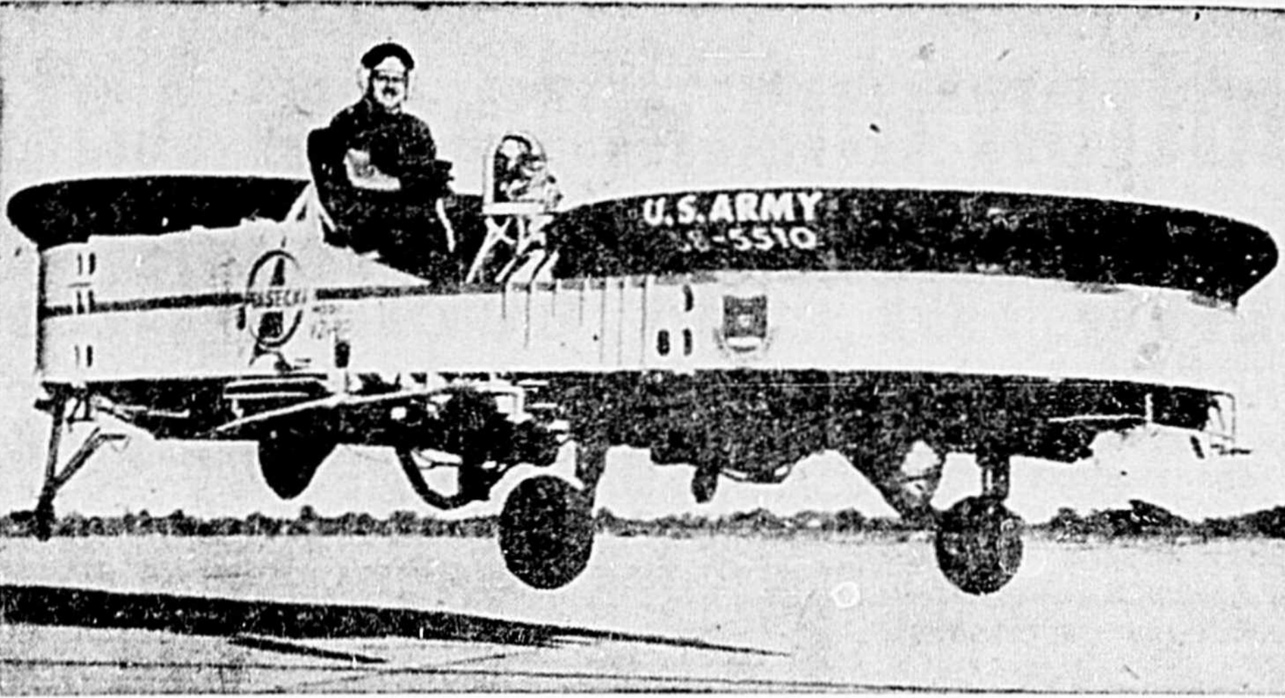
Voici la nouvelle voiture terrestre et partiellement aérienne de l'Armée américaine, le VZ-8F. Nous le voyons s'élever légèrement du terrain, lors de son premier essai. C'est le premier véhicule à pouvoir s'élever verticalement et voler, grâce à des appareils qui se trouvent à l'intérieur.
