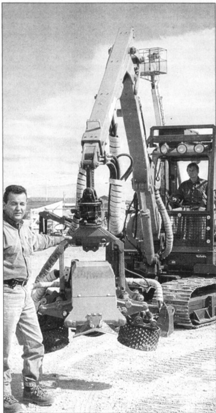
ABATTEUSE - Le travailleur forestier Guy Perron effectue ici quelques essais de routine avec le prototype d'abatteuse mis sur pied par l'entreprise CAM-TRAC sous les yeux du consultant Alain Savard.
