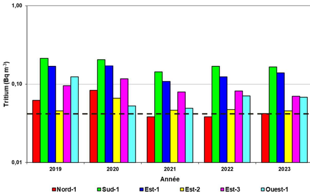
Figure 8-14 : Activité annuelle moyenne en tritium atmosphérique aux stations Nord-1, Sud-1, Est-1 à Est-3, Ouest-1 pour la période 2019-2023
