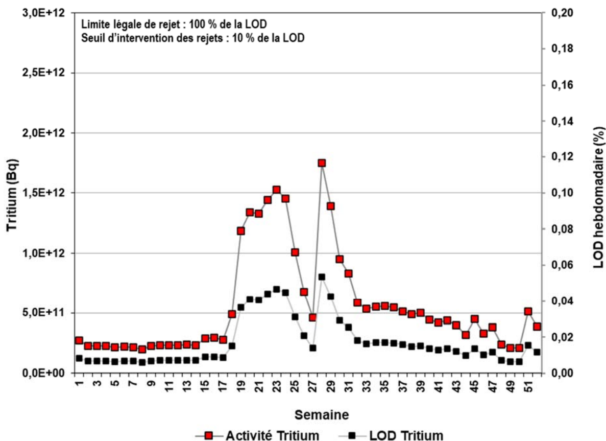
Figure 2-1 : Présence de tritium aux rejets gazeux de l'installation nucléaire de Gentilly-2, exprimée en % LOD et en activité sur une base hebdomadaire pour l'année 2023
