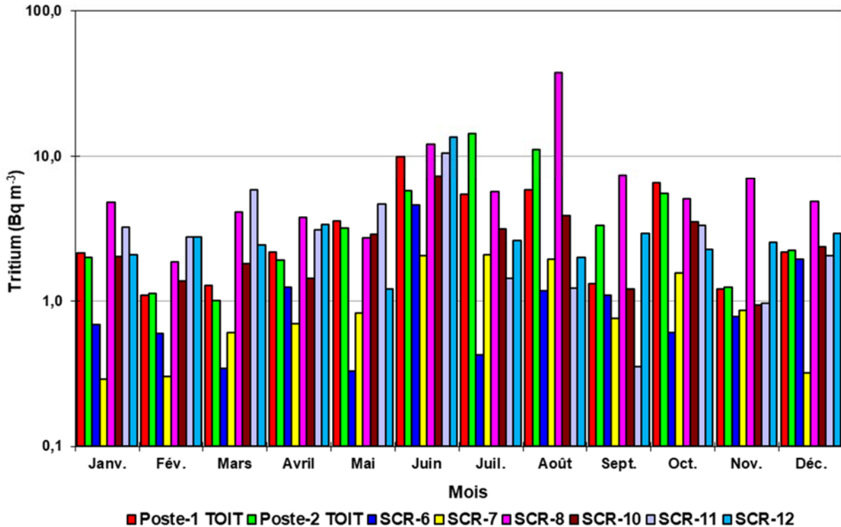
Figure 8-11 : Activité mensuelle en tritium atmosphérique aux stations Poste-1, Poste-2, SCR-6 à SCR-8 et SCR-10 à SCR-12 (zone d'exclusion) pour l'année 2023
