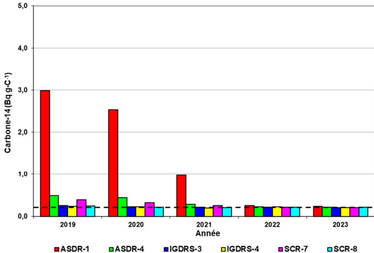
Figure 8-18 : Activité annuelle moyenne en carbone-14 atmosphérique aux stations IGDRS-3, IGDRS-4, ASDR-1, ASDR-4, SCR-7 et SCR-8 pour la période 2019-2023
