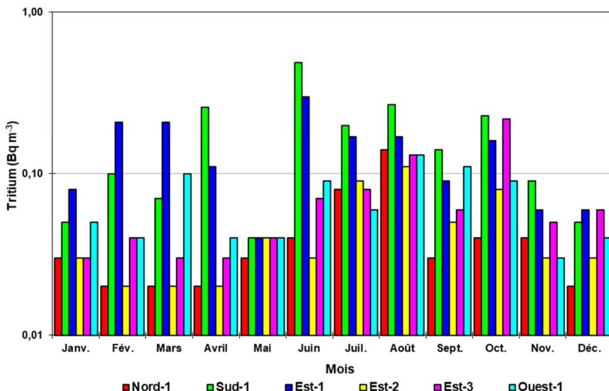
Figure 8-13 : Activité mensuelle en tritium atmosphérique aux stations Nord-1, Sud-1, Est-1 à Est-3, Ouest-1 et pour l'année 2023
