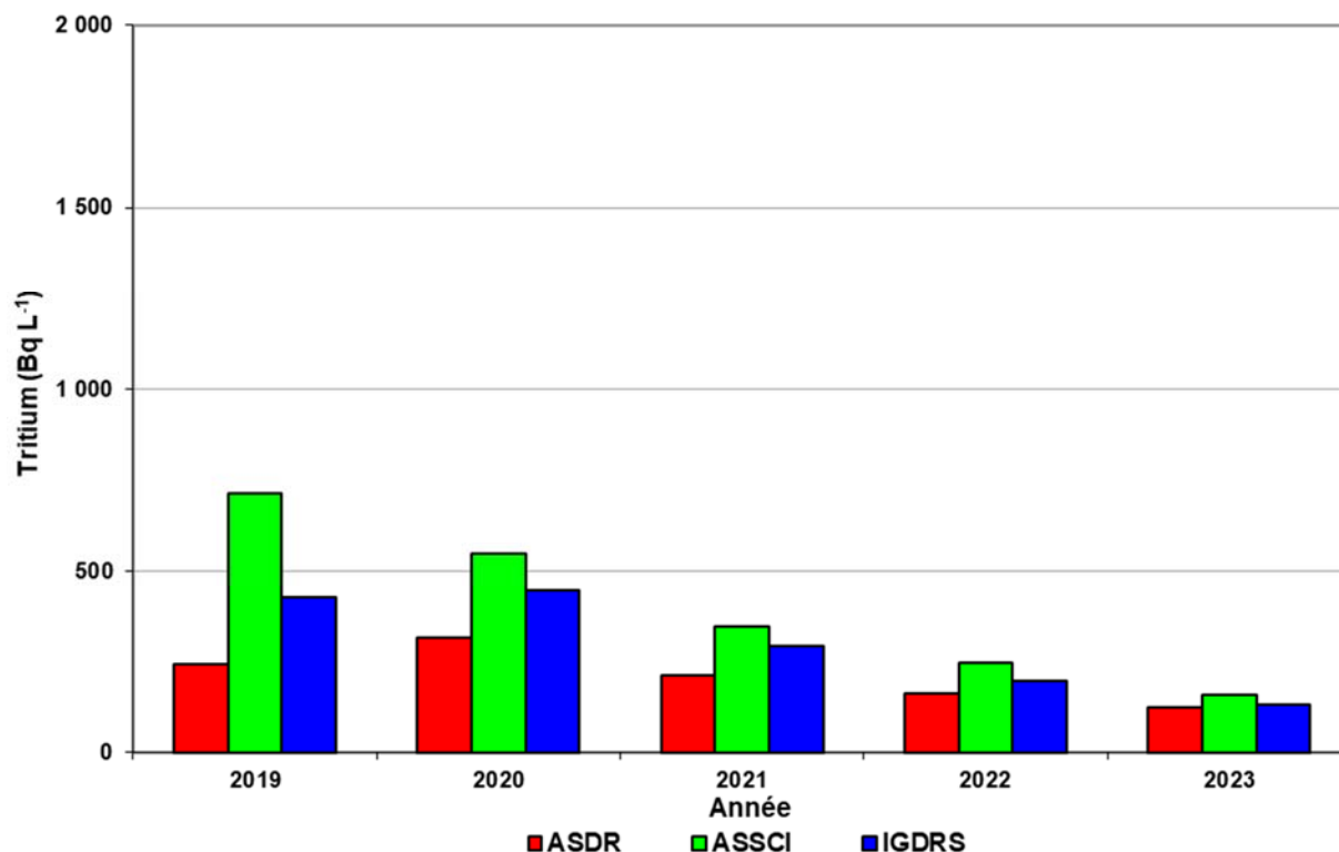
Figure 8-23 : Moyenne annuelle de l'activité en tritium dans l'eau de surface autour de l'ASDR, de l'ASSCI et de l'IGDRS pour la période 2019-2023
