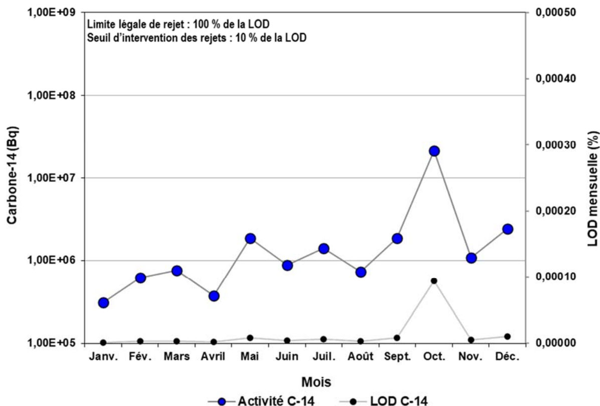
Figure 2-6 : Présence de carbone-14 aux effluents liquides de l'installation nucléaire de Gentilly-2, exprimée en % LOD et en activité sur une base mensuelle pour l'année 2023
