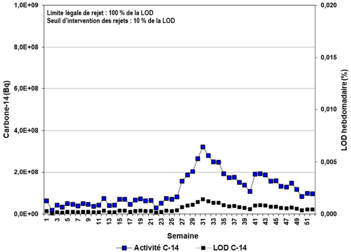
Figure 2-2 : Présence de carbone-14 aux rejets gazeux de l'installation nucléaire de Gentilly-2, exprimée en % LOD et en activité sur une base hebdomadaire pour l'année 2023
