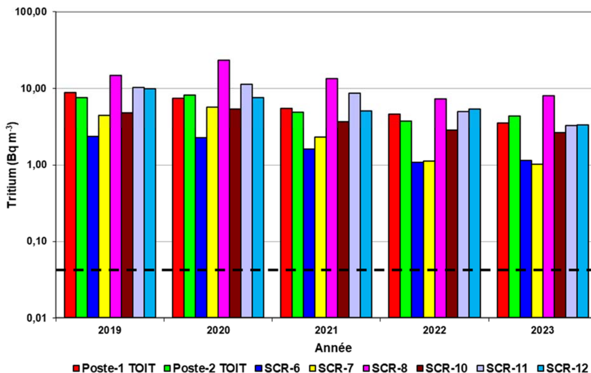
Figure 8-12 : Activité annuelle moyenne en tritium atmosphérique aux stations Poste-1, Poste-2, SCR-6 à SCR-8 et SCR-10 à SCR-12 (zone d'exclusion) pour la période 2019-2023
