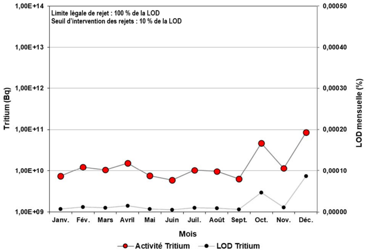
Figure 2-5 : Présence de tritium aux effluents liquides de l'installation nucléaire de Gentilly-2, exprimée en % LOD et en activité sur une base mensuelle pour l'année 2023
