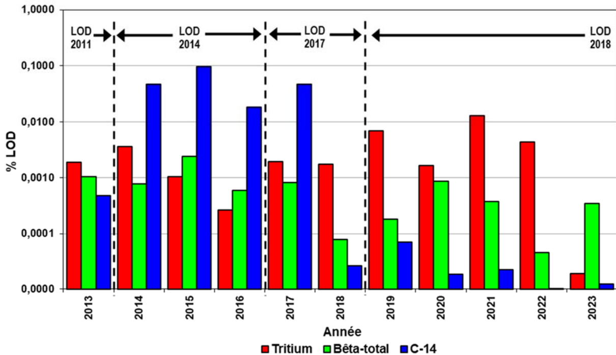
Figure 2-8 : Rejets radioactifs liquides annuels de l'installation nucléaire de Gentilly-2 exprimés en % LOD pour la période 2013-2023
