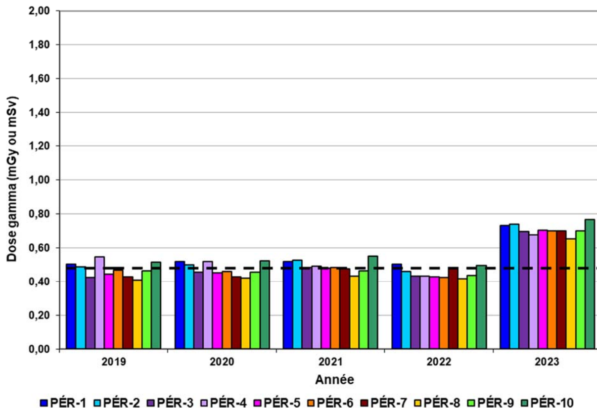
Figure 8-4 : Dose annuelle gamma au périmètre sécurisé de l'installation pour la période 2019-2023
