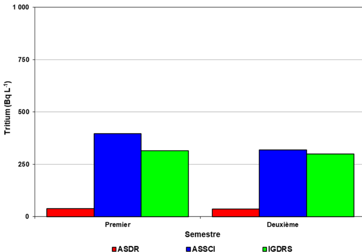
Figure 8-28 : Moyenne semestrielle de l'activité en tritium dans l'eau souterraine de l'ASDR, de l'ASSCI et de l'IGDRS pour l'année 2023
