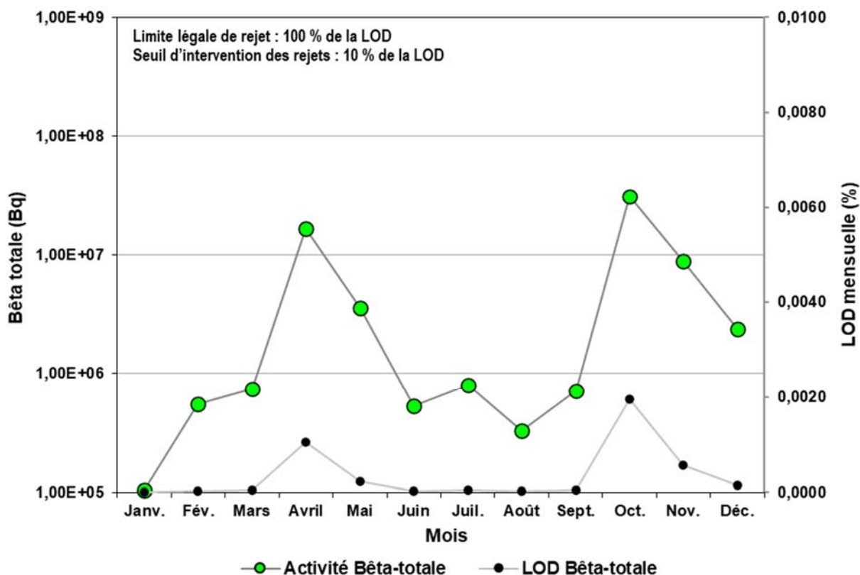
Figure 2-7 : Présence d'activité bêta totale aux effluents liquides de l'installation nucléaire de Gentilly-2, exprimée en % LOD et en activité sur une base mensuelle pour l'année 2023
