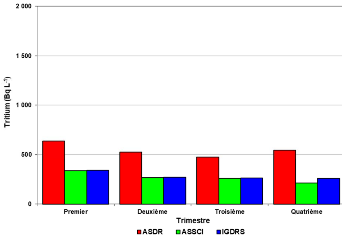
Figure 8-25 : Moyenne trimestrielle de l'activité en tritium dans l'eau d'infiltration autour de l'ASDR, de l'ASSCI et de l'IGDRS pour l'année 2023
