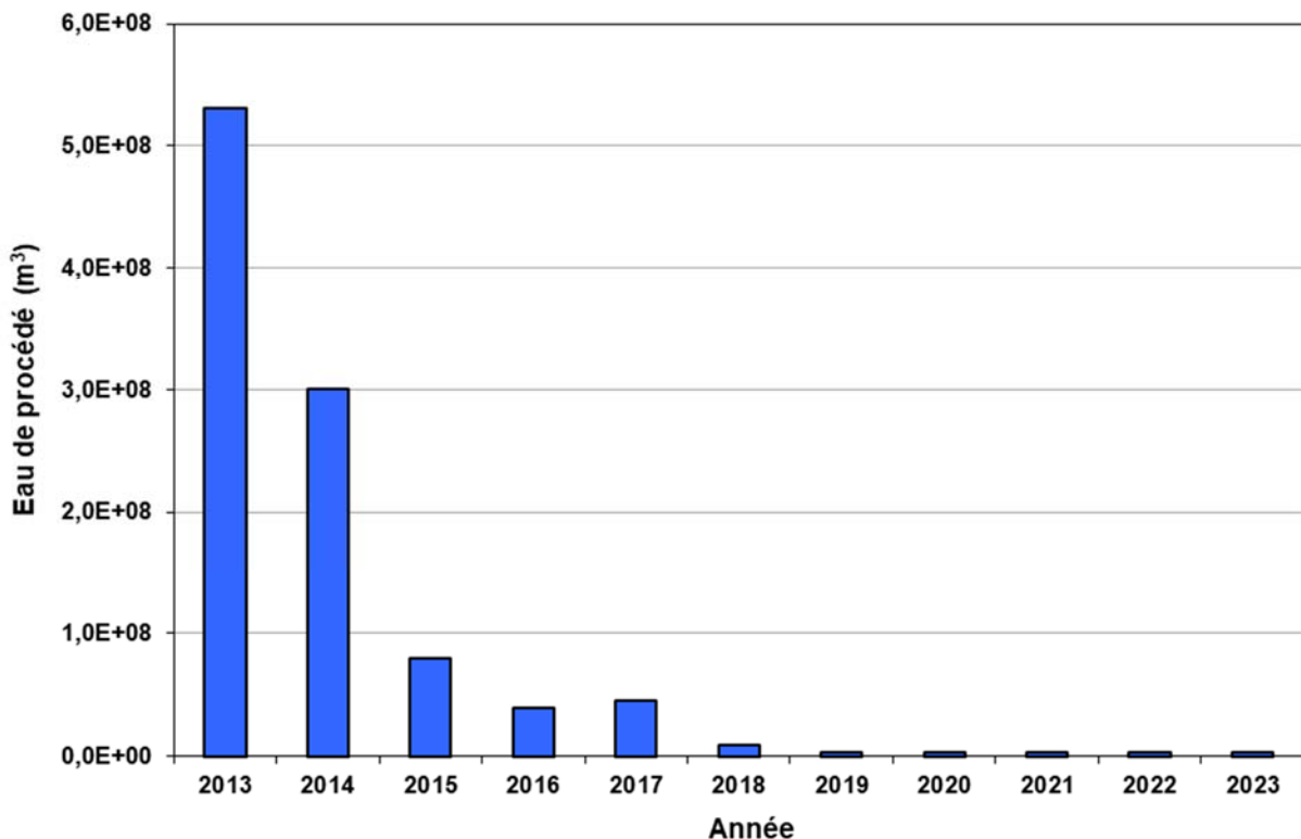
Figure 5-1 : Consommation d'eau de procédé aux installations de Gentilly-2 pour la période 2013-2023
