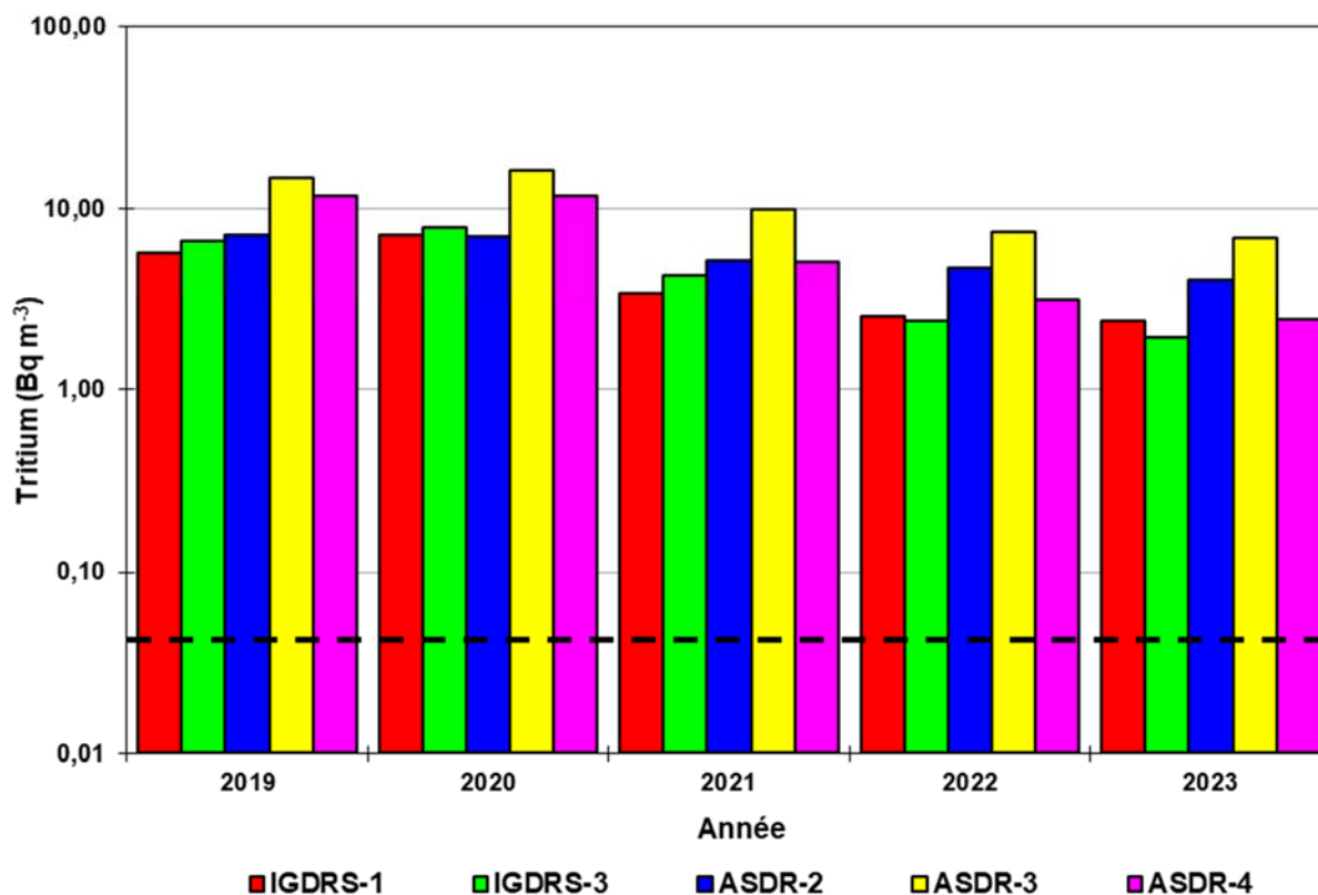
Figure 8-16 : Activité annuelle moyenne de tritium atmosphérique à l'IGDRS et l'ASDR pour la période 2019-2023
