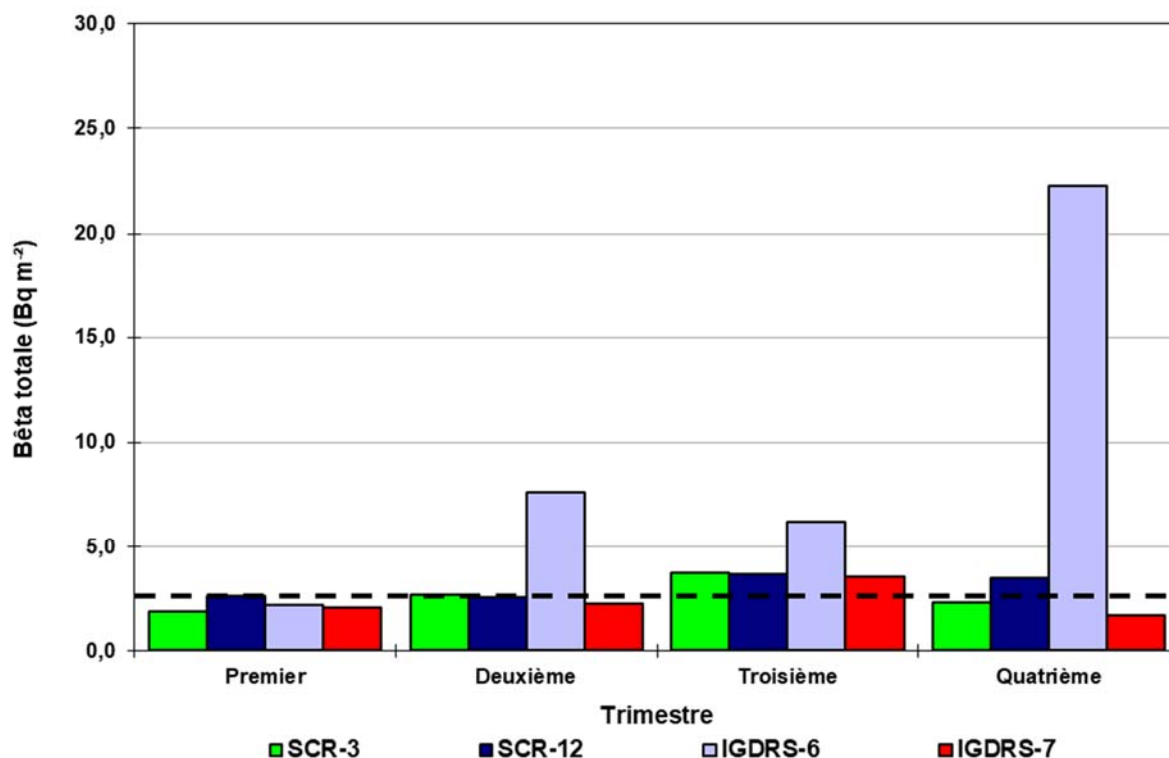
Figure 8-21 : Moyenne trimestrielle de l'activité bêta totale dans les précipitations aux stations SCR-3, SCR-12, IGDRS-6 et IGDRS-7 pour l'année 2023
