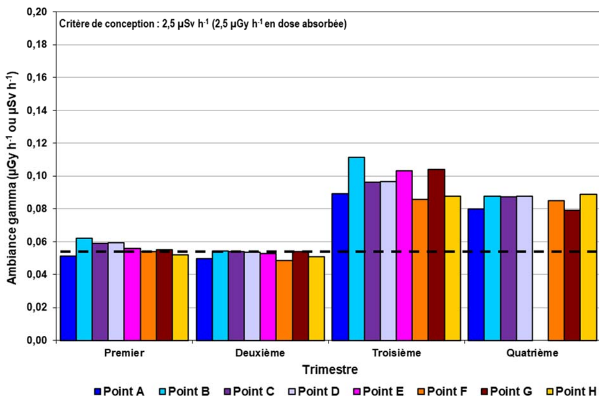
Figure 8-5 : Ambiance gamma trimestrielle à la clôture de l'ASDR pour l'année 2023
