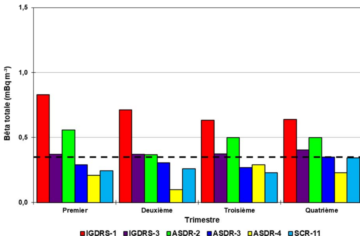
Figure 8-19 : Moyenne trimestrielle de l'activité bêta totale dans les aérosols prélevés aux stations IGDRS-1, IGDRS-3, ASDR-2, ASDR-3, ASDR-4 et SCR-11 pour l'année 2023
