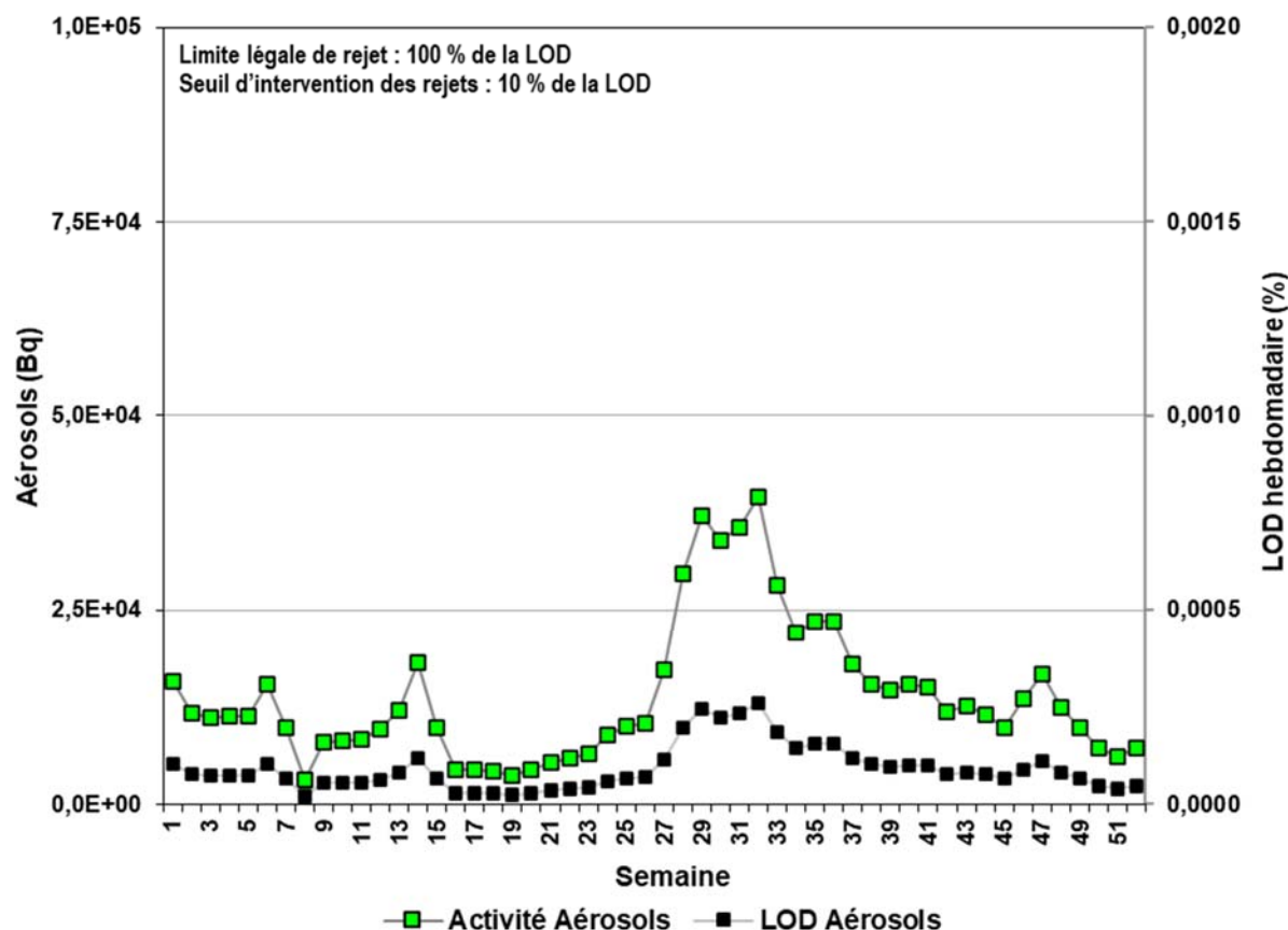
Figure 2-3 : Présence d'aérosols radioactifs aux rejets gazeux de l'installation nucléaire de Gentilly-2, exprimée en % LOD et en activité sur une base hebdomadaire pour l'année 2023
