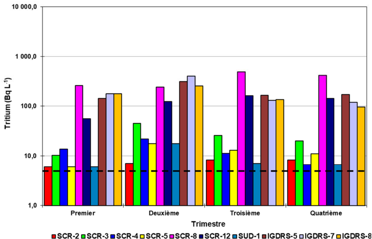
Figure 8-20 : Moyenne trimestrielle de l'activité en tritium dans les précipitations aux stations SCR-2 à SCR-5, SCR-8, SCR-12, Sud-1, IGDRS-5, IGDRS-7 et IGDRS-8 pour l'année 2023
