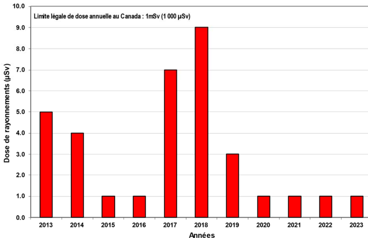
Figure 9-1 : Dose annuelle de rayonnements estimée pour un membre représentatif de la population liée au déclassement des installations de Gentilly-2 pour la période 2013-2023
