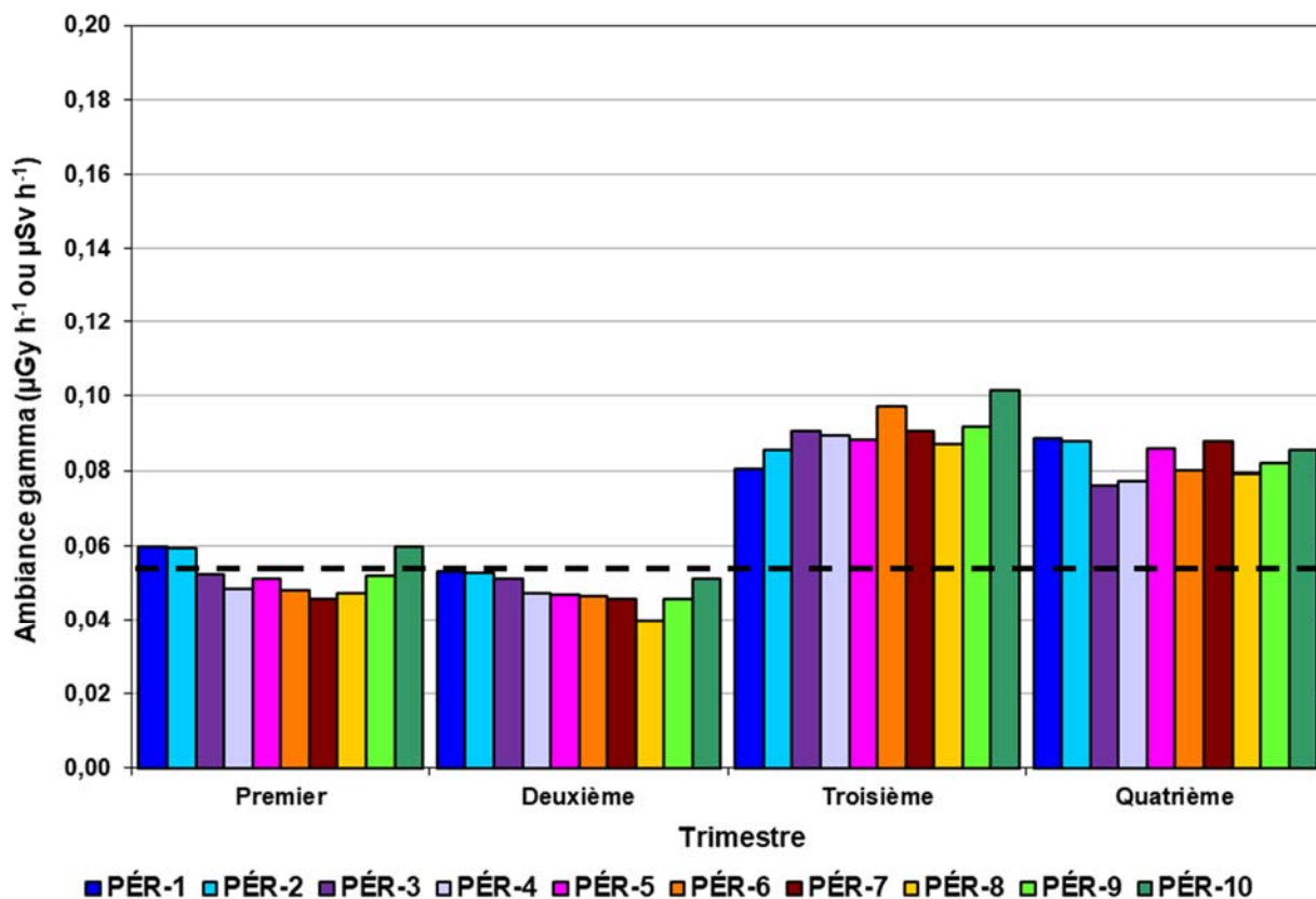
Figure 8-3 : Ambiance gamma trimestrielle au périmètre sécurisé de l'installation pour l'année 2023
