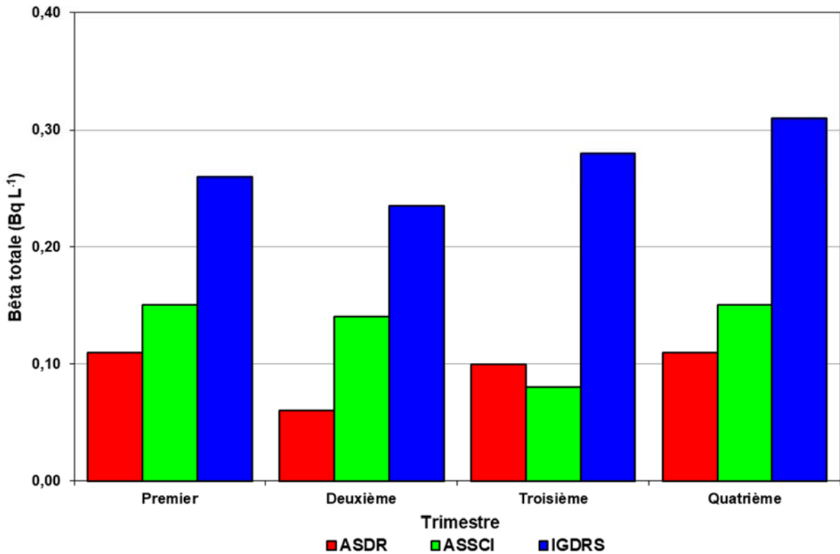
Figure 8-27 : Moyenne trimestrielle de l'activité bêta totale dans l'eau d'infiltration autour de l'ASDR, de l'ASSCI et de l'IGDRS pour l'année 2023
