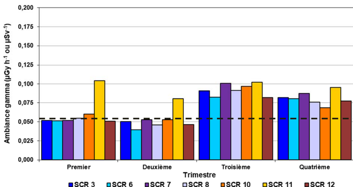
Figure 8-1 : Ambiance gamma trimestrielle aux stations de contrôle SCR-3, 6, 7, 8, 10, 11 et 12 (zone rapprochée) pour l'année 2023
