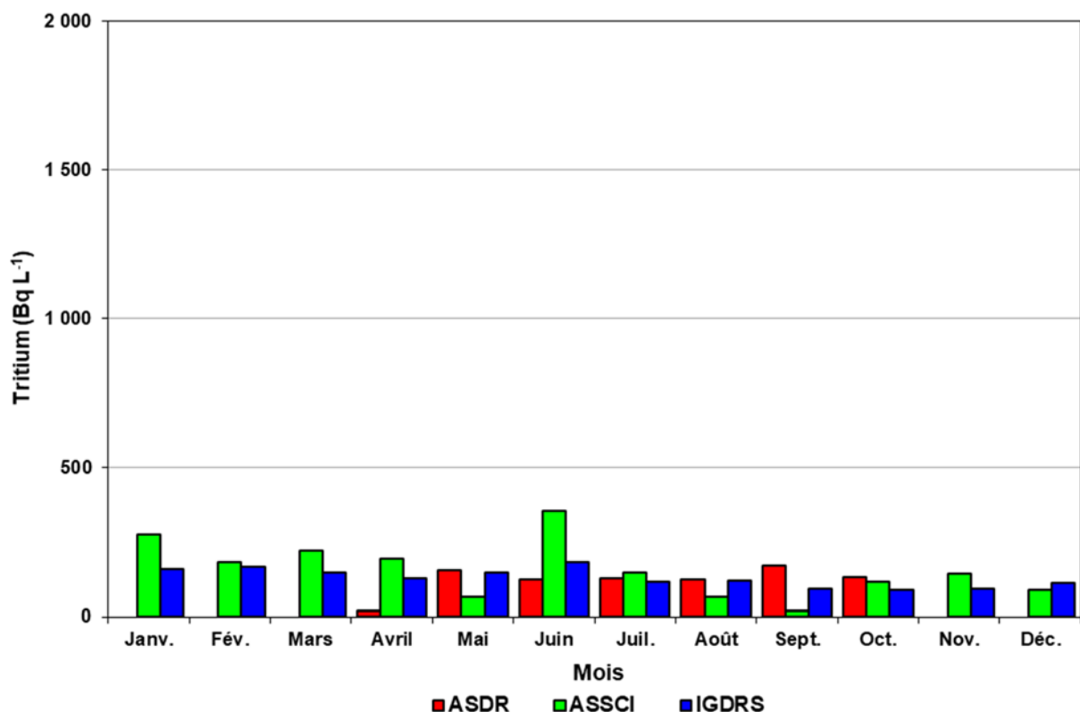
Figure 8-22 : Moyenne mensuelle de l'activité en tritium dans l'eau de surface autour de l'ASDR, de l'ASSCI et de l'IGDRS pour l'année 2023
