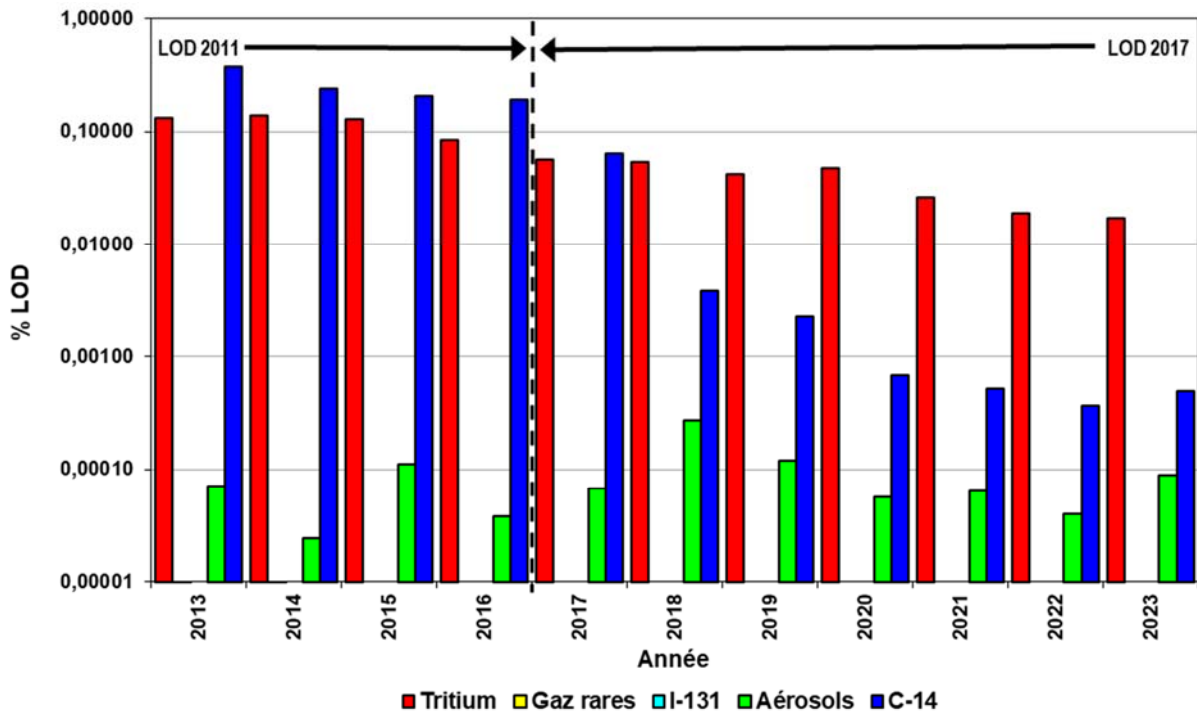
Figure 2-4 : Rejets radioactifs gazeux annuels de l'installation nucléaire de Gentilly-2 exprimés en % LOD pour la période 2013-2023
