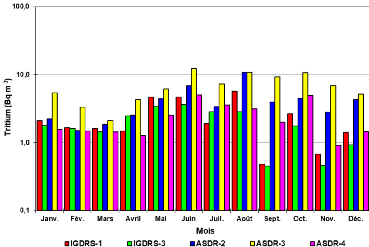
Figure 8-15 : Activité mensuelle en tritium atmosphérique à l'IGDRS et l'ASDR pour l'année 2023
