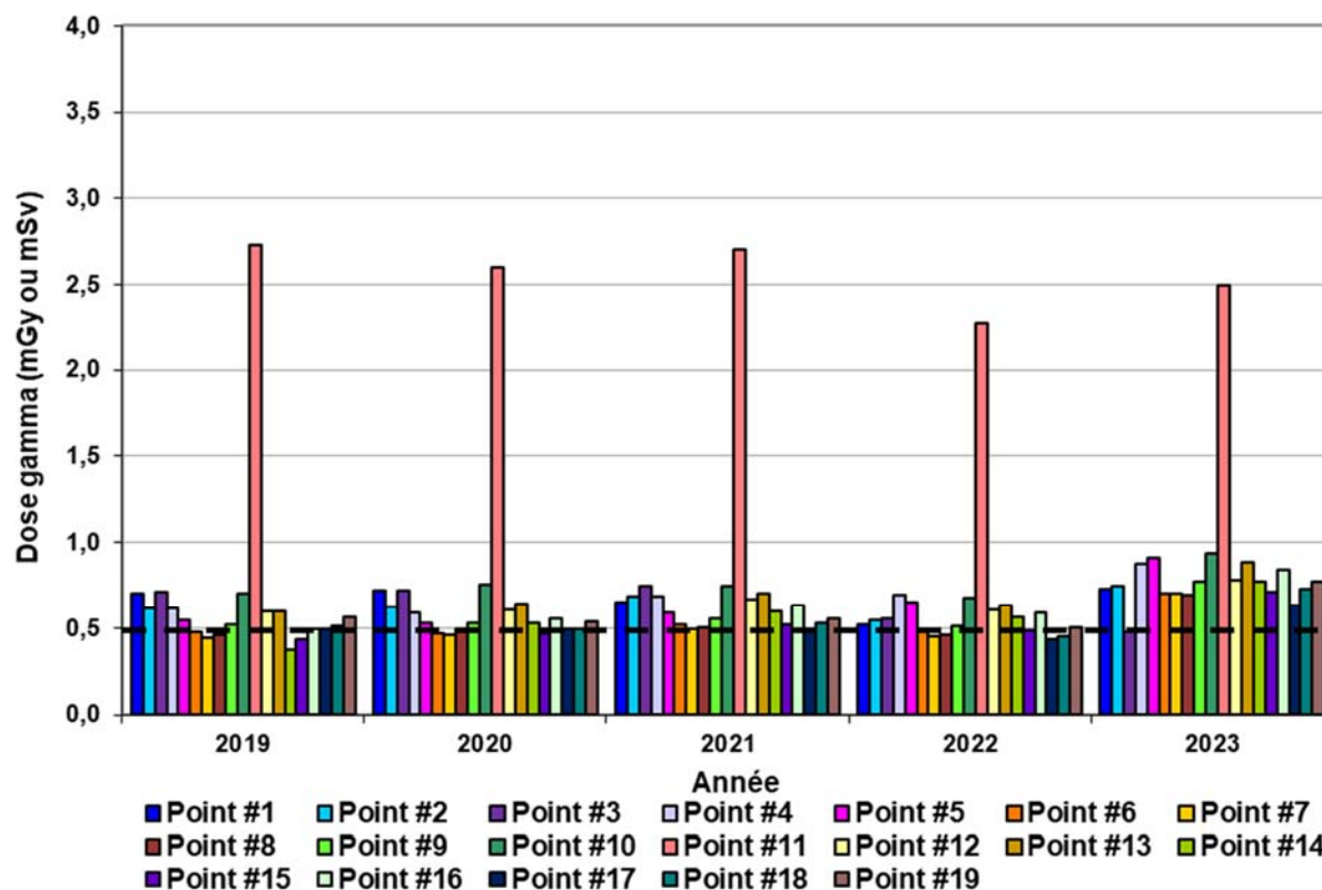
Figure 8-8 : Dose annuelle gamma à la clôture de l'IGDRS pour la période 2019-2023
