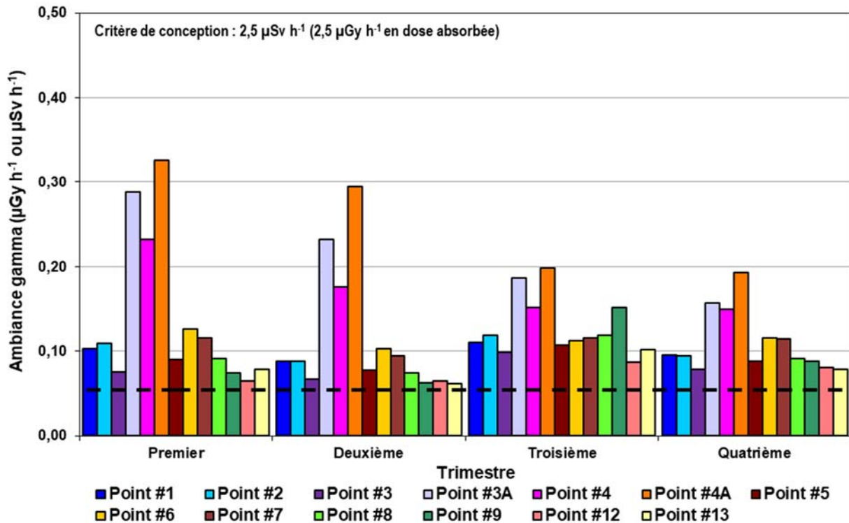
Figure 8-9 : Ambiance gamma trimestrielle à la clôture de l'ASSCI pour l'année 2023
