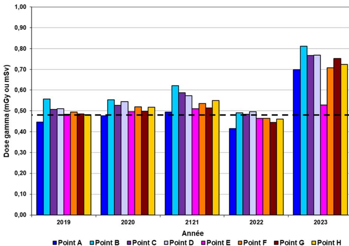
Figure 8-6 : Dose annuelle gamma à la clôture de l'ASDR pour la période 2019-2023
