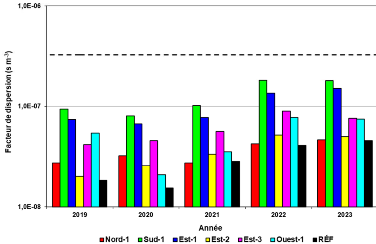
Figure 8-35 : Facteurs moyens de dispersion du tritium atmosphérique des relâches des installations de Gentilly-2 pour la période 2019-2023
