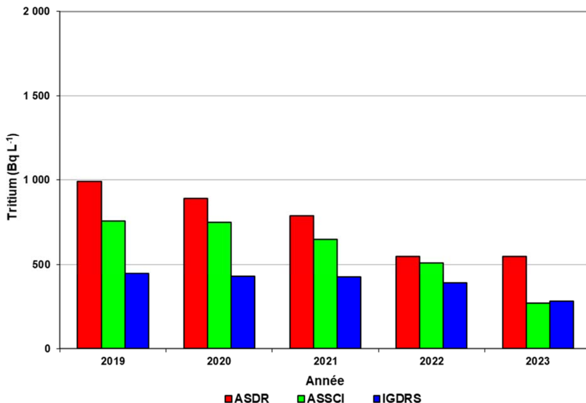
Figure 8-26 : Moyenne annuelle de l'activité en tritium dans l'eau d'infiltration autour de l'ASDR, de l'ASSCI et de l'IGDRS pour la période 2019-2023
