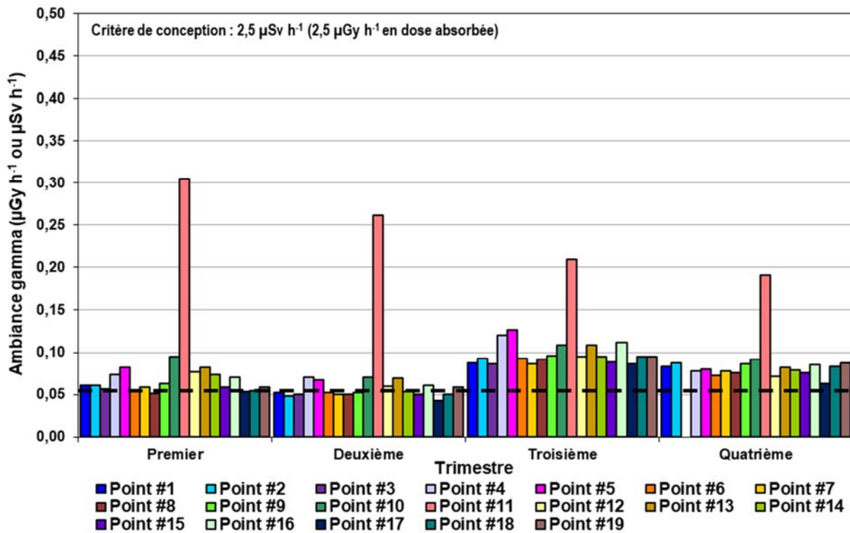
Figure 8-7 : Ambiance gamma trimestrielle à la clôture de l'IGDRS pour l'année 2023
