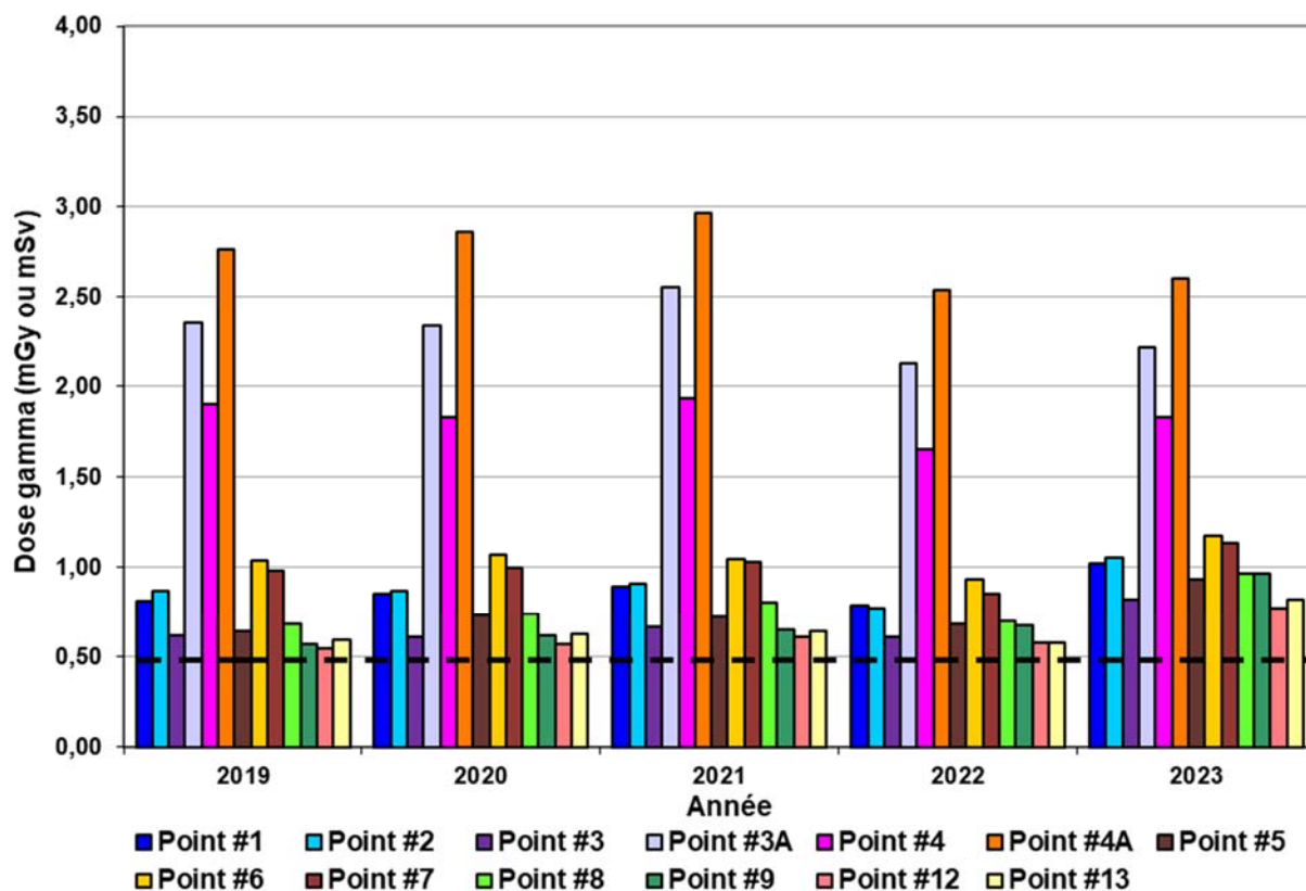
Figure 8-10 : Dose annuelle gamma à la clôture de l'ASSCI pour la période 2019-2023
