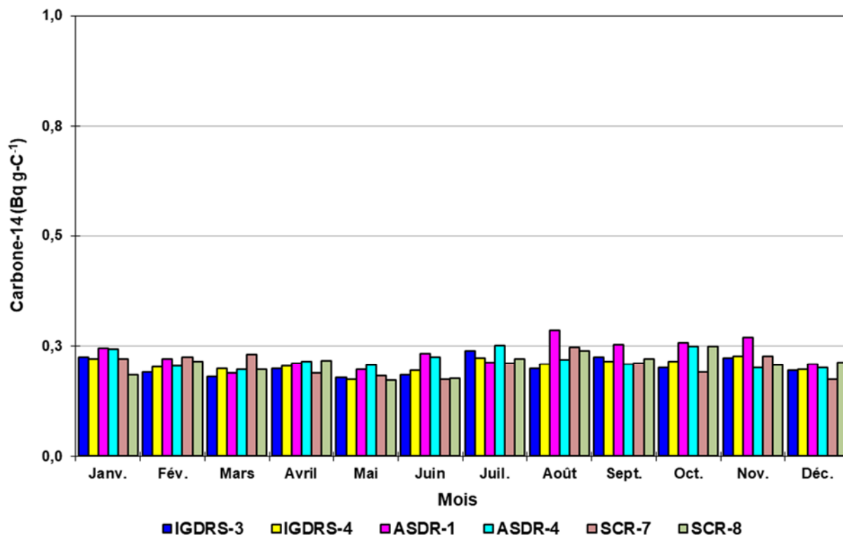
Figure 8-17 : Activité mensuelle en carbone-14 atmosphérique aux stations IGDRS-3, IGDRS-4, ASDR-1, ASDR-4, SCR-7 et SCR-8 pour l'année 2023
