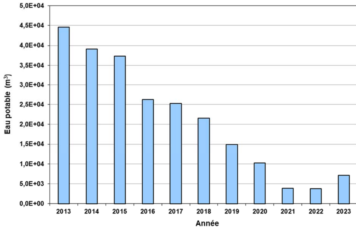
Figure 5-2 : Consommation d'eau potable aux installations de Gentilly-2 pour la période 2013-2023
