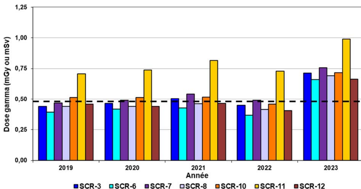
Figure 8-2 : Dose annuelle gamma aux stations de contrôle SCR-3, 6, 7, 8, 10, 11 et 12 (zone rapprochée) pour la période 2019-2023
