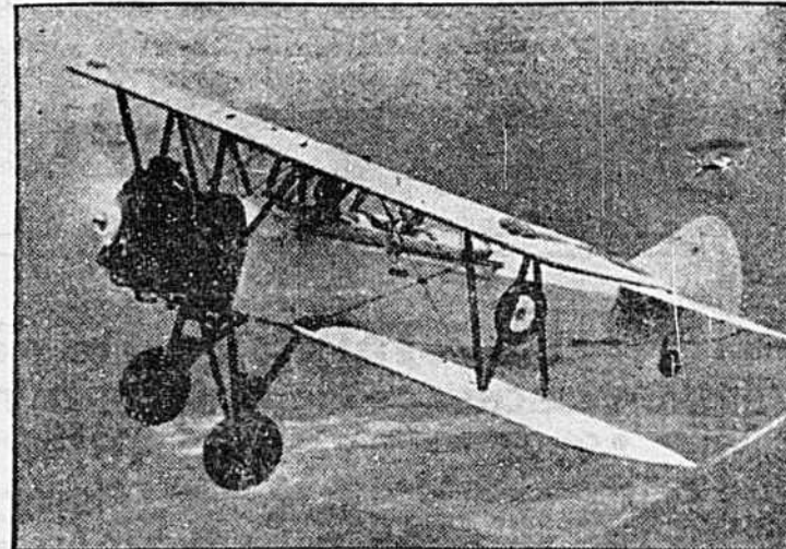
"Le Fleet Finch", un biplan à deux places dont il est fait usage pour apprendre le pilotage aux recrues de l'Aviation royale du Canada dans les écoles élémentaires d'entraînement aérien. Cet avion a une vitesse limitée à 165 milles à l'heure et son unique moteur a une force de 125 h.p. seulement.
