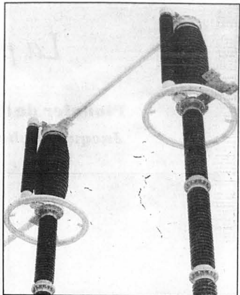
Le disjoncteur GFX Grand Froid, tel qu'on aura bientôt l'occasion de le voir sur les lignes de haute tension.
