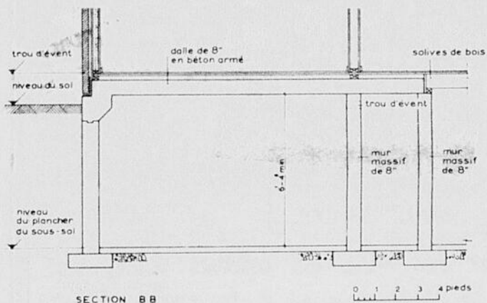
Ce dessin illustre une section longitudinale de l'abri où la hauteur de six pieds quatre pouces est le strict minimum.
