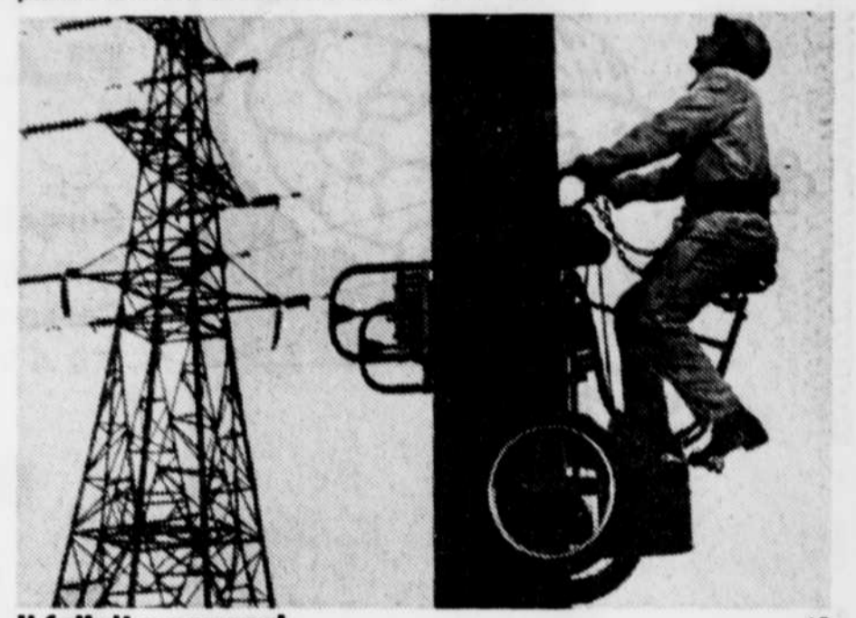
Il fallait y penser! Un ingénieur soviétique a inventé un engin à pédales qui permet aux techniciens de grimper au sommet des pylônes électriques en béton pour installer ou réparer des câbles. Cette bicyclette verticale est munie de bras qui ensèrent le pylône tandis que l'ouvrier actionne les roues qui lui permettent de monter ou de descendre. Une licence de production a déjà été vendue à l'Allemagne de l'Est.
