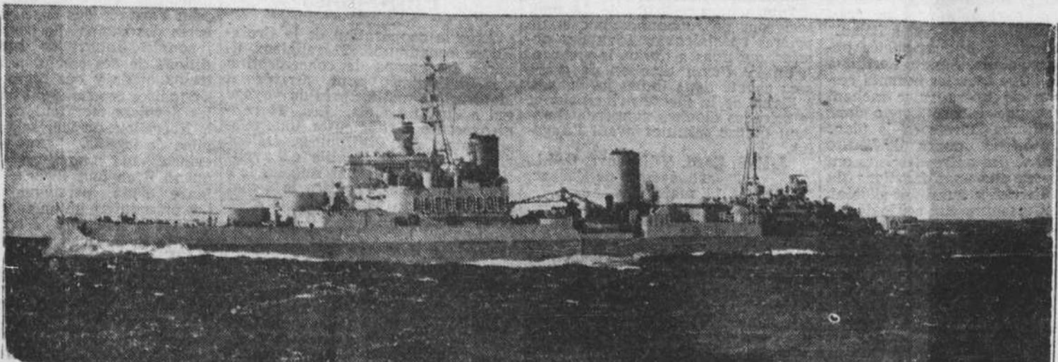
C'est en 1944 que la Marine royale canadienne se procura un premier croiseur moderne, l'"Ouganda". Le beau navire, qui déplace 8,000 tonnes et possède un armement principal de neuf canons de six pouces, est actuellement en service dans le Pacifique. (Photo de la Marine royale canadienne)
