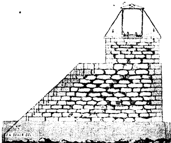
Echafaudage pour la construction d'un tube.
