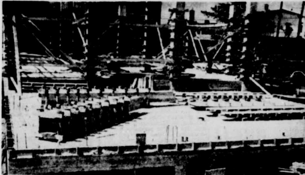
Shawinigan-Sud, 8. (DNC). — Les travaux de la salle municipale de Shawinigan-Sud vont bon train sous la direction de M. A. C. Fleischman. On voit ici les fondations de béton armé qui sont terminées tandis que on est à élever les formes pour couler les piliers qui supporteront le rez-de-
