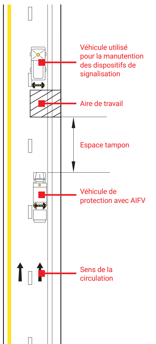
SCHEMA AVEC VEHICULE DE PROTECTION MUNI D'UN AIFV
