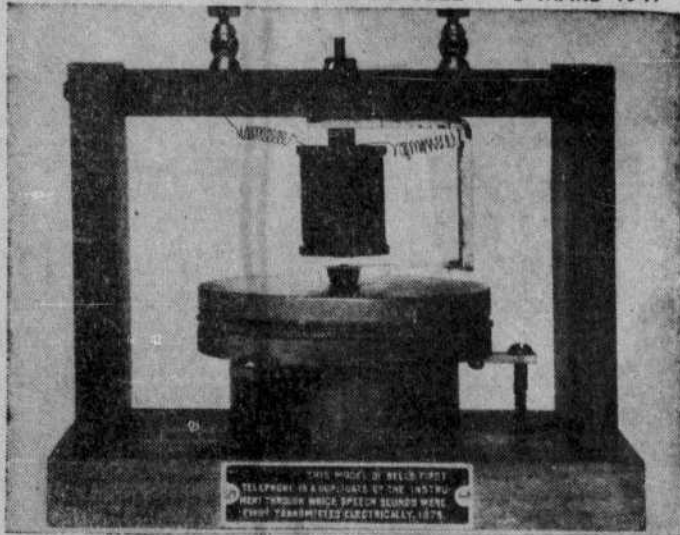
Voici une réplique du premier appareil téléphonique utilisé pour la transmission de la voix. Un alimant attaché à un diaphragme de boudruche produisait un courant ondulatoire dans la bobine. C'est sur ce même principe que repose le fonctionnement des téléphones dont sont munis certains navires de guerre.
