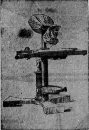
Voici une réplique du premier appareil téléphonique utilisé pour la transmission de la voix. Un alimant attaché à un diaphragme de boudruche produisait un courant ondulatoire dans la bobine. C'est sur ce même principe que repose le fonctionnement des téléphones dont sont munis certains navires de guerre.
