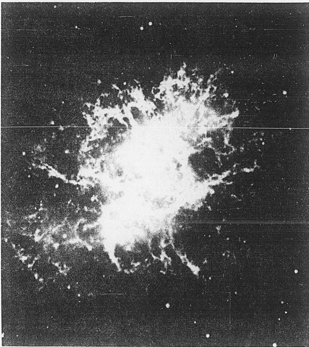
La nébuleuse du Crabe est ce qui reste d'une explosion stellaire enregistrée par les astronomes chinois en 1056 de notre ère. Des recherches récentes semblent indiquer qu'une importante explosion stellaire survenue il y a des milliers d'années a pu influencer sur l'évolution de la vie sur Terre, et sur la vie de l'homme.
