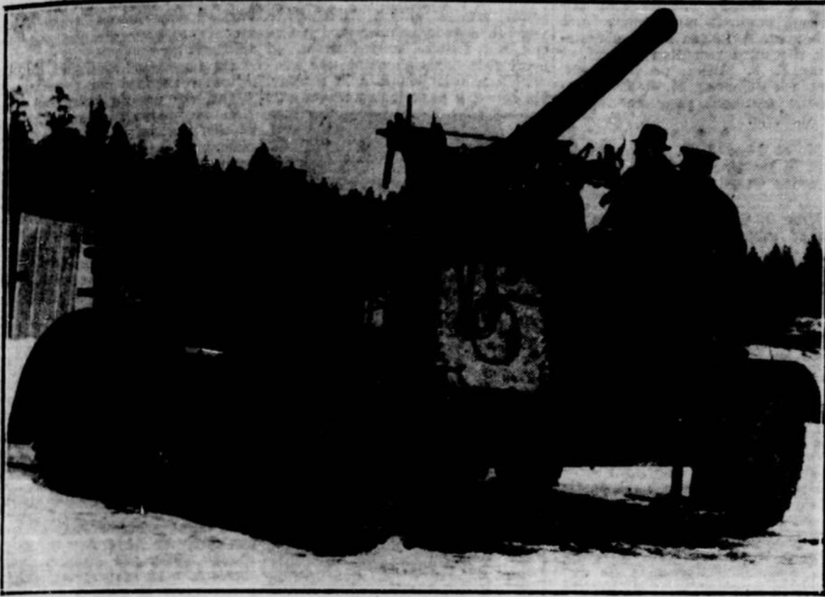
CELUI-CI TIRE SEUL. — Relié électriquement à un merveilleux télémètre qu'il nous a été impossible de photographier, voici un canon contre avions capable de tirer sans servants. Seul, l'observateur au télémètre peut déclencher le tir d'une simple pression du doigt. (Photo de l'envoyé du "Petit Journal").
