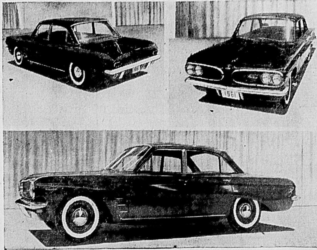
Voici trois illustrations de la Tempest 1961, la nouvelle voiture à moteur quatre cylindres lancée au Canada par Pontiac. C'est la première voiture du continent nord-américain munie d'un moteur à l'avant et d'une boîte de vitesses à l'arrière. Pontiac a conçu le moteur de la Tempest en adoptant son moteur V-8, moins les cylindres du côté gauche.
