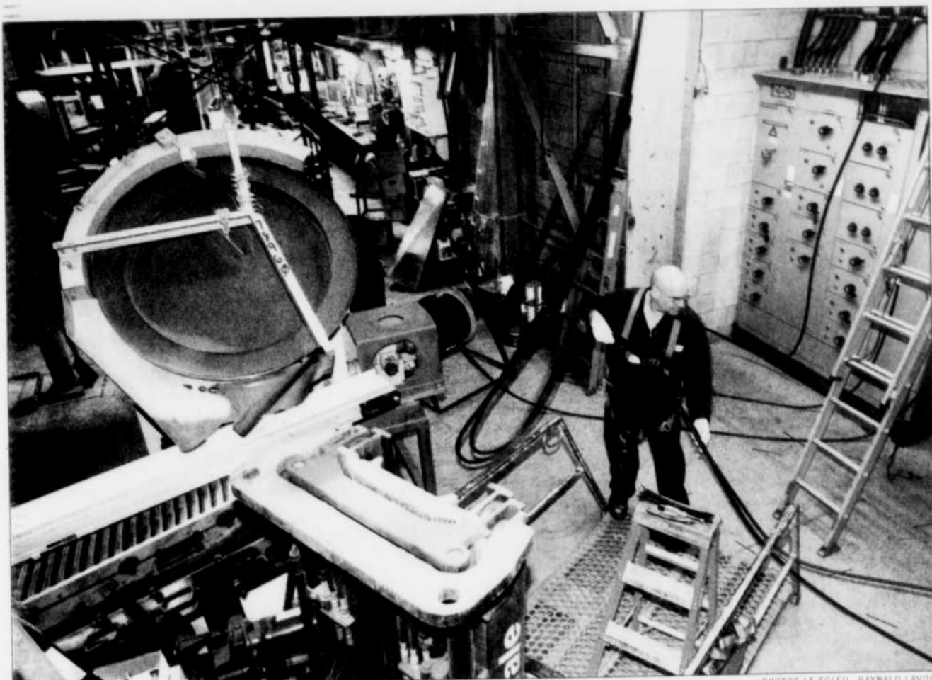
Le technicien Michel Lachance est en train d'installer dans l'usine-laboratoire un nouvel équipement de simulation d'une valeur de 1 million $. Il servira à valider une nouvelle méthode de cuisson des boulettes de minerai de fer.
