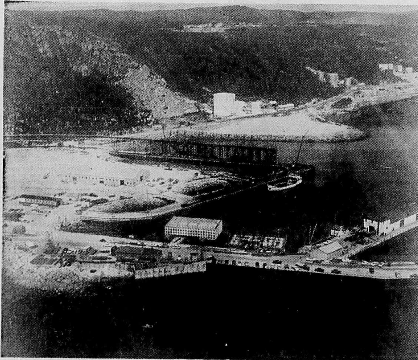
Ces nouvelles facilités portuaires comprennent deux nouveaux quais. La structure neuve genre de brise-eau construit le long du quai, puis transporté et partiellement immergé dans le port.
