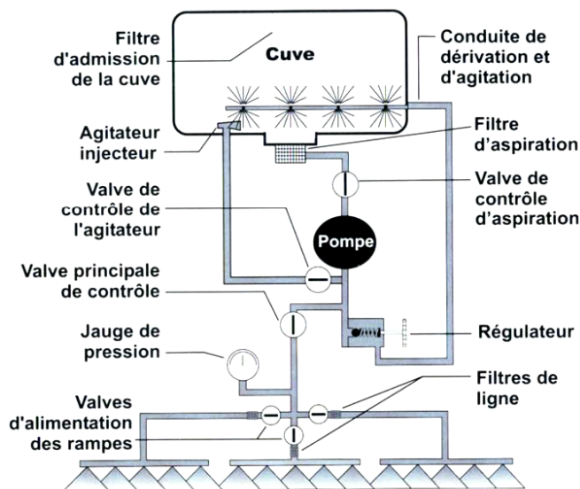
Schéma d'un pulvérisateur à rampe
