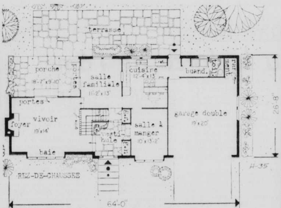
PLAN DES DEUX ETAGES — Sans tenir compte du garage, de l'aire de service et des porches, ce plan bien agencé totalise 1,974 pieds carrés — 965 pieds carrés au rez-de-chaussée et 1,009 pieds carrés à l'étage supérieur. Les dimensions hors tout sont de 64' de longueur sur 26' 8" de largeur.
