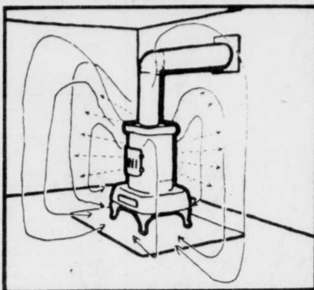
La chaleur, à partir d'un poêle, se répand dans la pièce par rayonnement et par convection. Il est possible de chauffer partiellement une pièce adjacente par l'aménagement de registres pratiqués dans la cloison et en tenant la porte ouverte.
