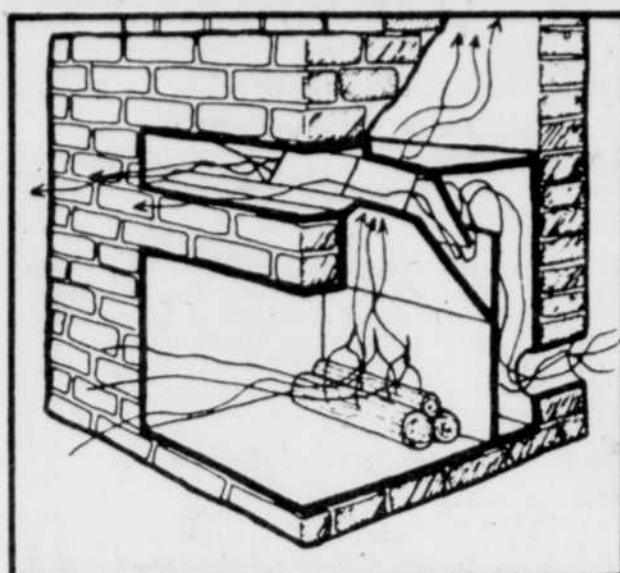
Le foyer à circulation d'air typique: l'air peut être très chaud dans les conduits, qui ne doivent pas être connectés aux conduits d'air froid d'une fournaise existante. D'où forte déperdition de chaleur.
