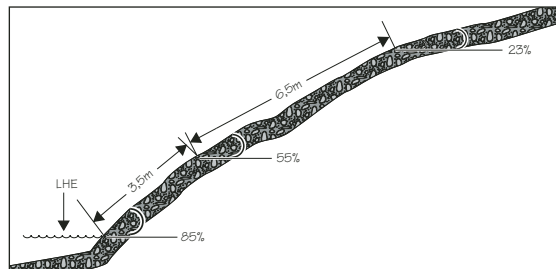
Figure 52 : Le talus comporte des changements de pente
