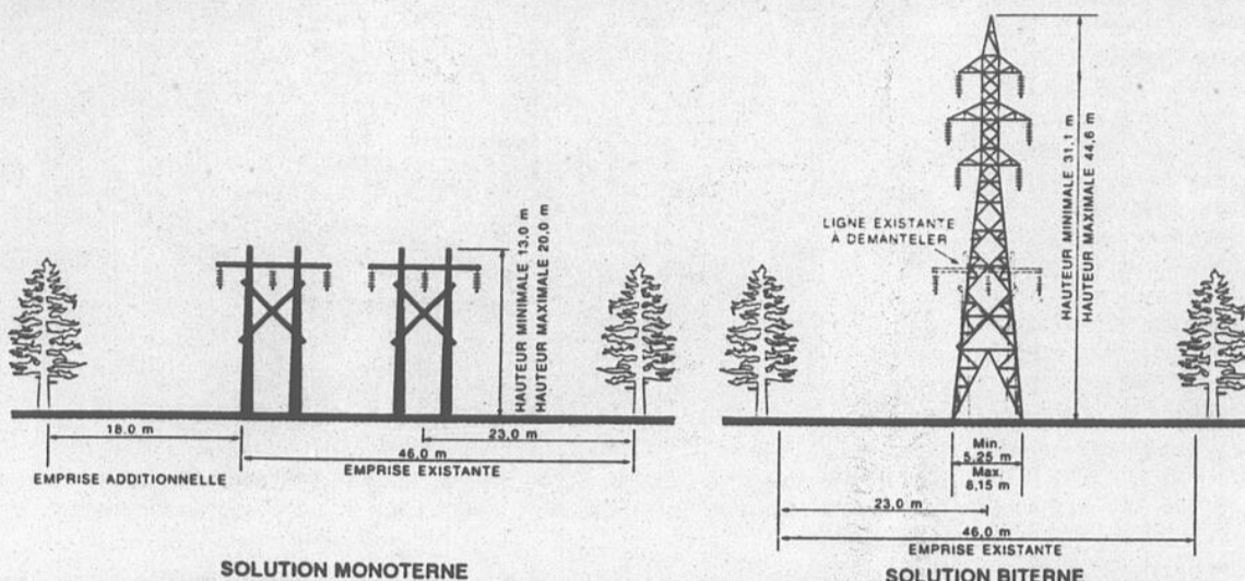
Un aperçu des solutions monoterne et biterne. La première exige un élargissement de l'emprise actuel pour l'ajout d'une deuxième ligne alors que la solution numéro deux consiste au démantèlement de la ligne existante afin de permettre l'installation d'une nouvelle ligne sur pylône en treillis métalliques qui présentent l'inconvénient d'être deux fois plus élevés que les pylônes de bois. Ils s'intègrent donc plus difficilement au paysage.
