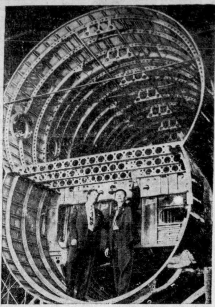
On voit ici le fuselage d'un avion de transport géant "Boeing", à deux étages, que l'on est en train de construire actuellement dans une usine de Seattle. Ce géant des airs accommodera 55 passagers, leur fournissant des lits, des salons, et un bar où ils pourront prendre des consommations.
