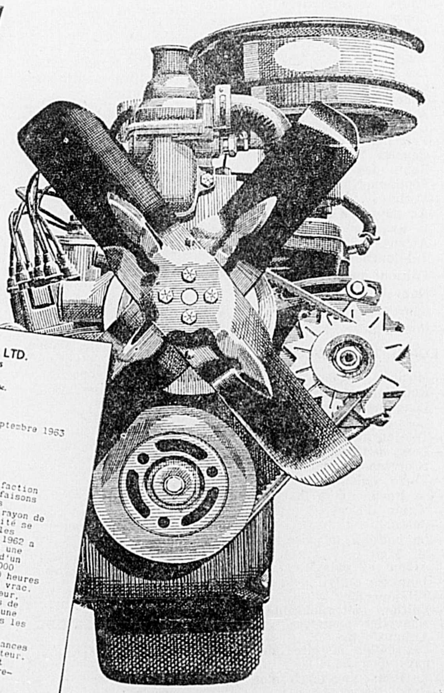
Le six-cyl. 292: un des moteurs de camions 1964, éprouvés à la tâche.
