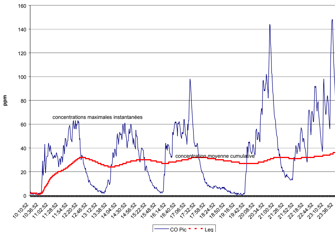
Figure 1 : Concentrations ambiantes de CO lors d'une compétition de motocross dans l'aréna de Val-d'Or en 1999 (doté d'un système de ventilation par dilution d'air)
