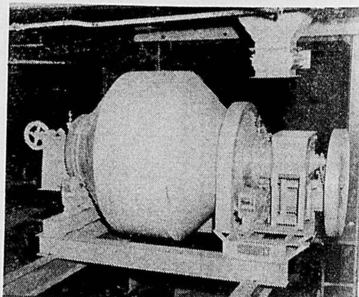
Malaxeur hautement spécialisé servant au mélange des micro-ingrédients.
