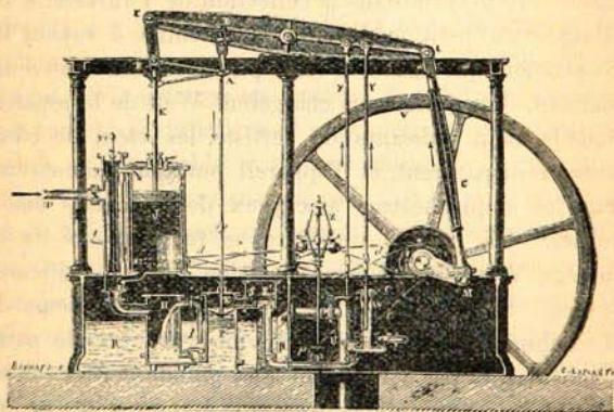
MACHINE A BALANCIER.
