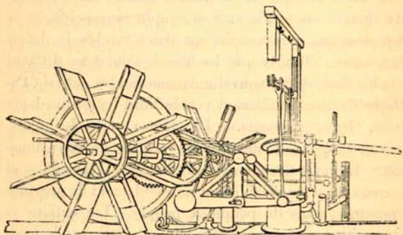
Les Machines du "Clermont" fabriquées en Angleterre; diamètre des roues 15 pieds, et le cylindre 24 pouces de diamètre.
