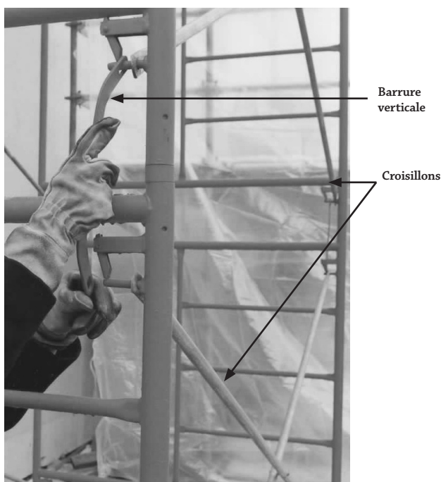
Contreventement d'un échafaudage sur cadres métalliques
