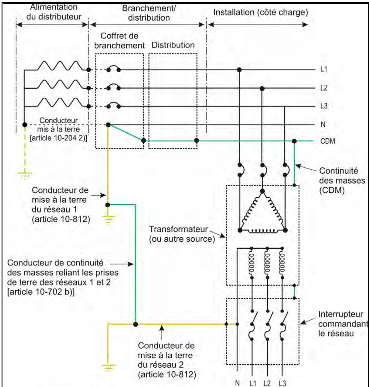
Figure 4 MALT indépendante des réseaux interreliés par CDM (à l'interrupteur)
