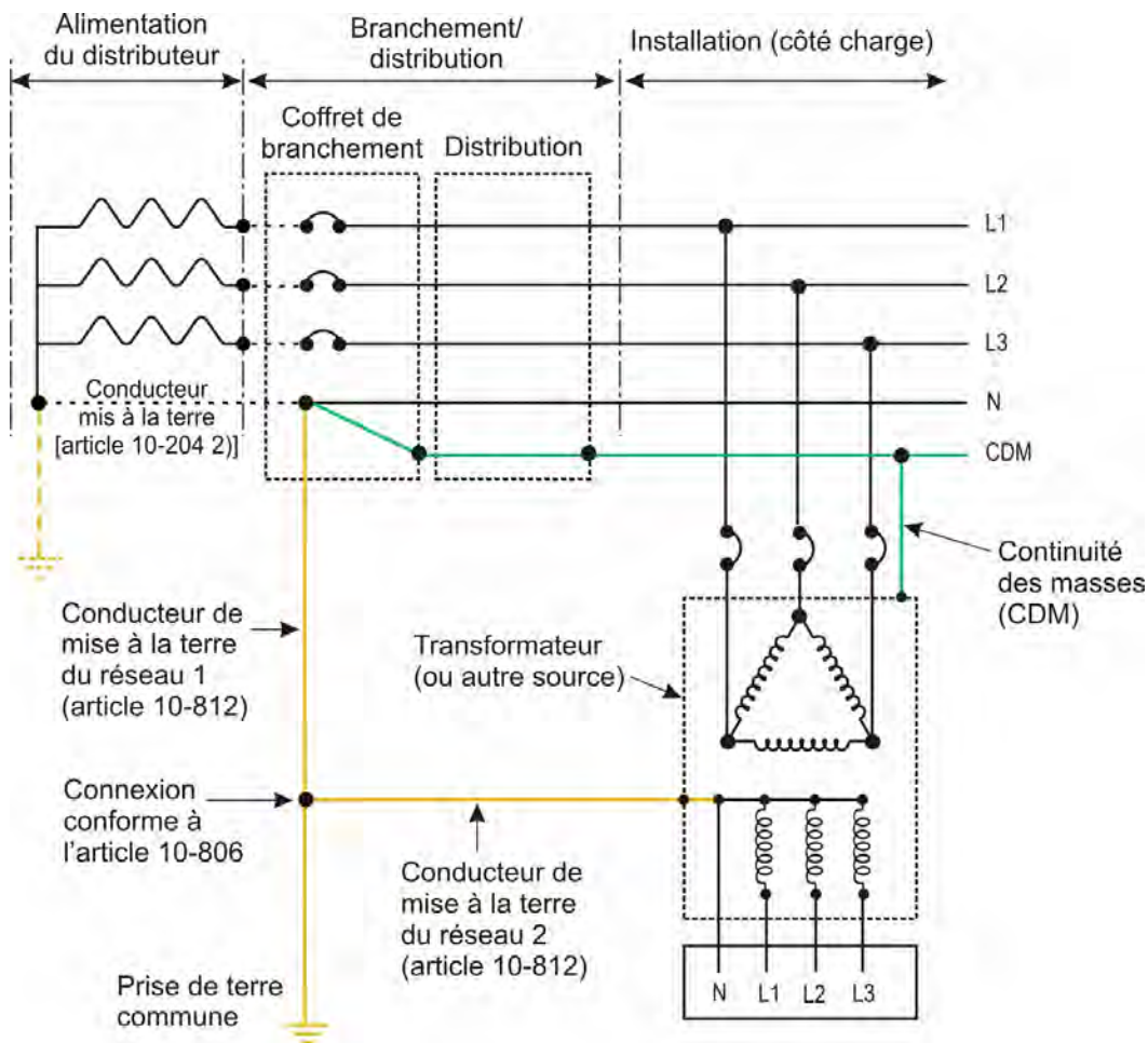
Figure 1 MALT commune des réseaux
